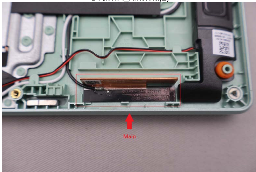
BT&amp;WIFI_Antenna(2)
