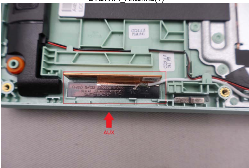
BT&amp;WIFI_Antenna(1)
