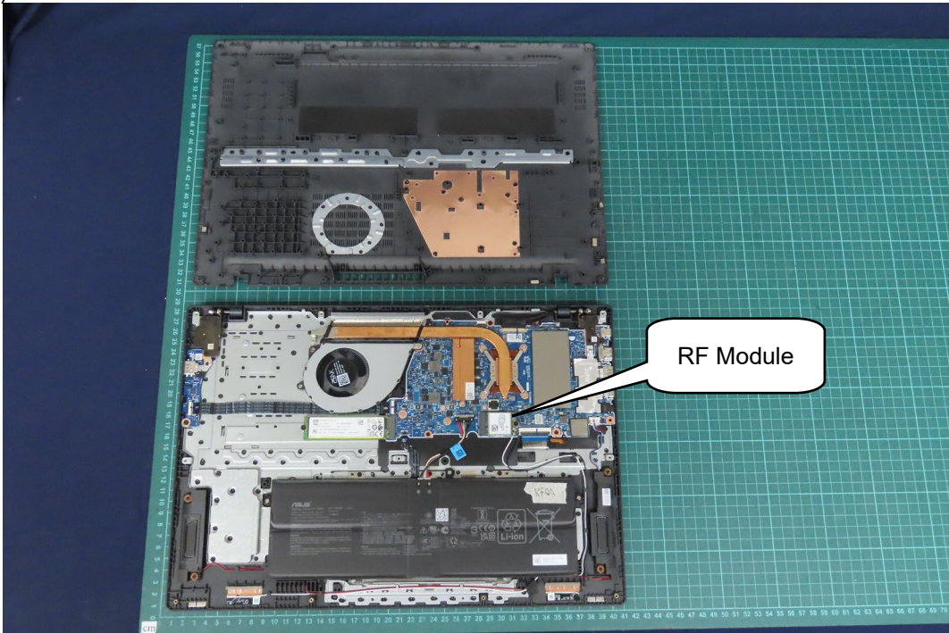
(13)EUT Photo
