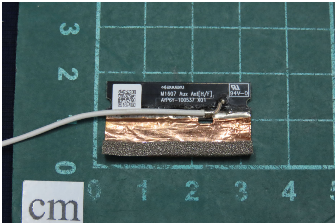
(10) EUT Photo
