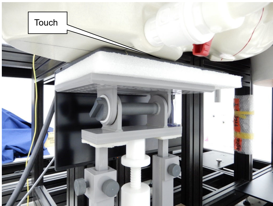
EUT Bottom of laptop_Ant Aux
