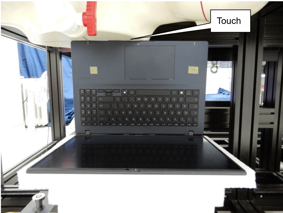
EUT Front edge of laptop_Ant Aux
