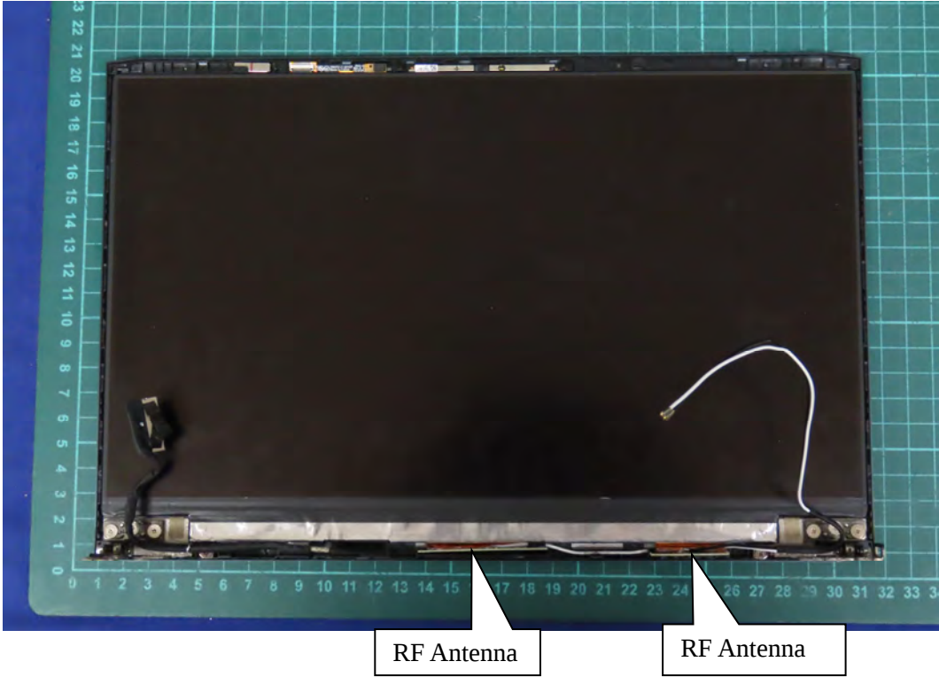
(24) EUT Photo
