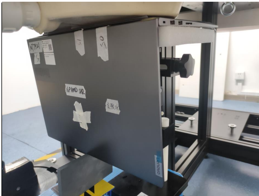
Bottom Side (0mm) Aux. Antenna
