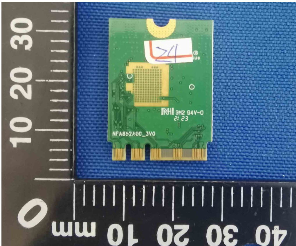
RF MODULE BACK VIEW_RTL8852BE
