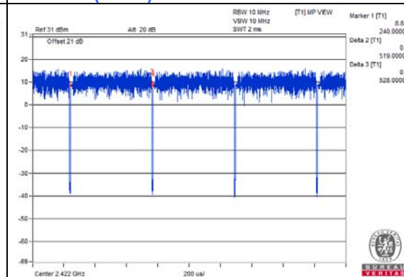
802.11ax (RU52)
