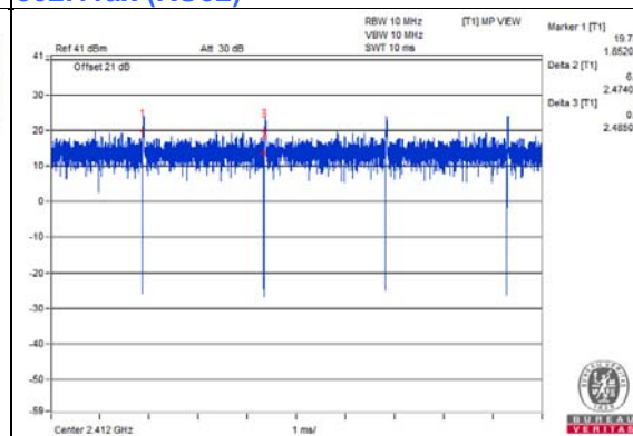
802.11ax (RU52)
