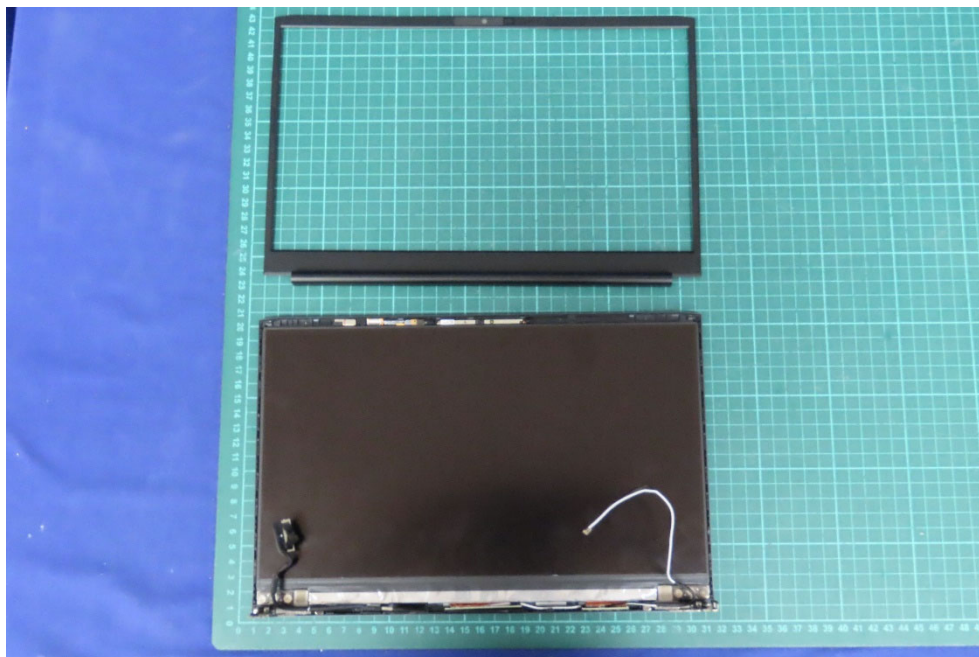
(30) EUT Photo
