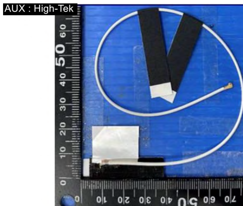
EUT Photo (14)
