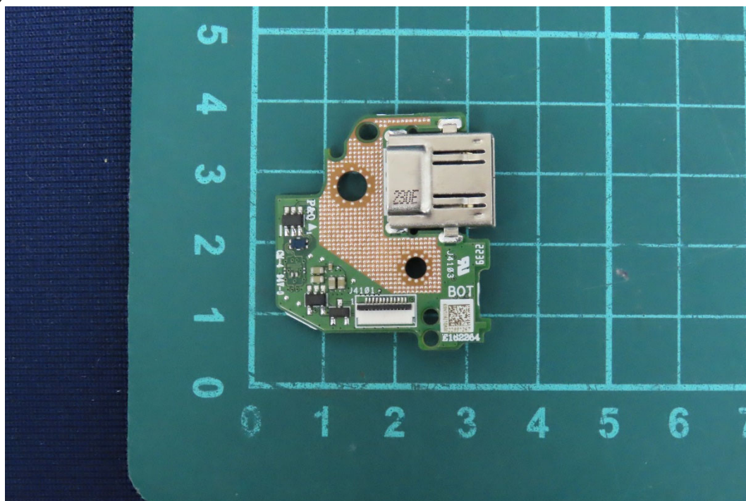
(20) EUT Photo
