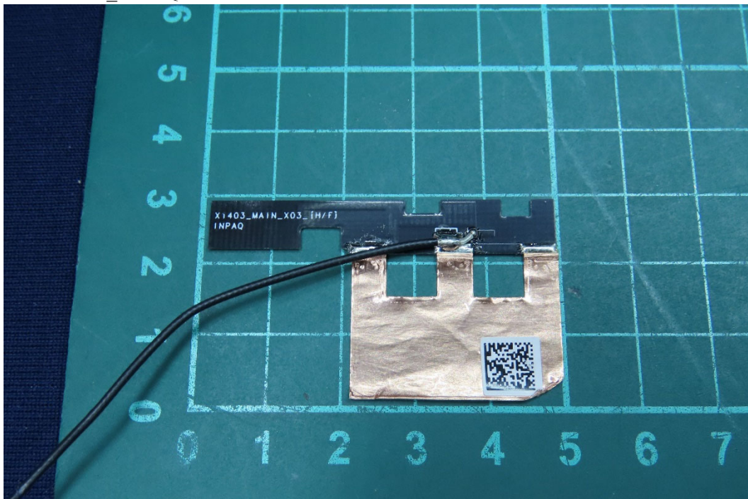
(27) EUT Photo_INPAQ Main Antenna
