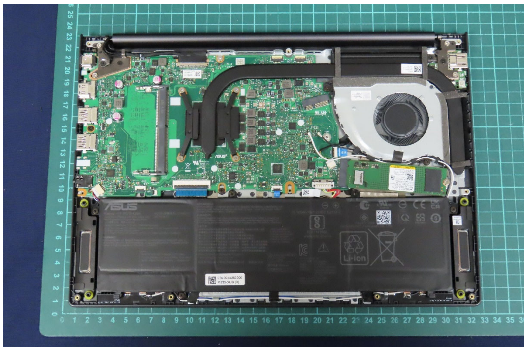
(13) EUT Photo
