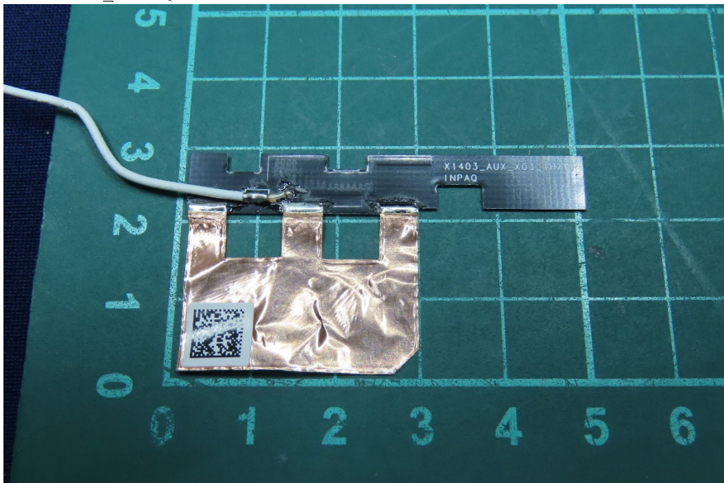
(29) EUT Photo_INPAQ Aux Antenna
