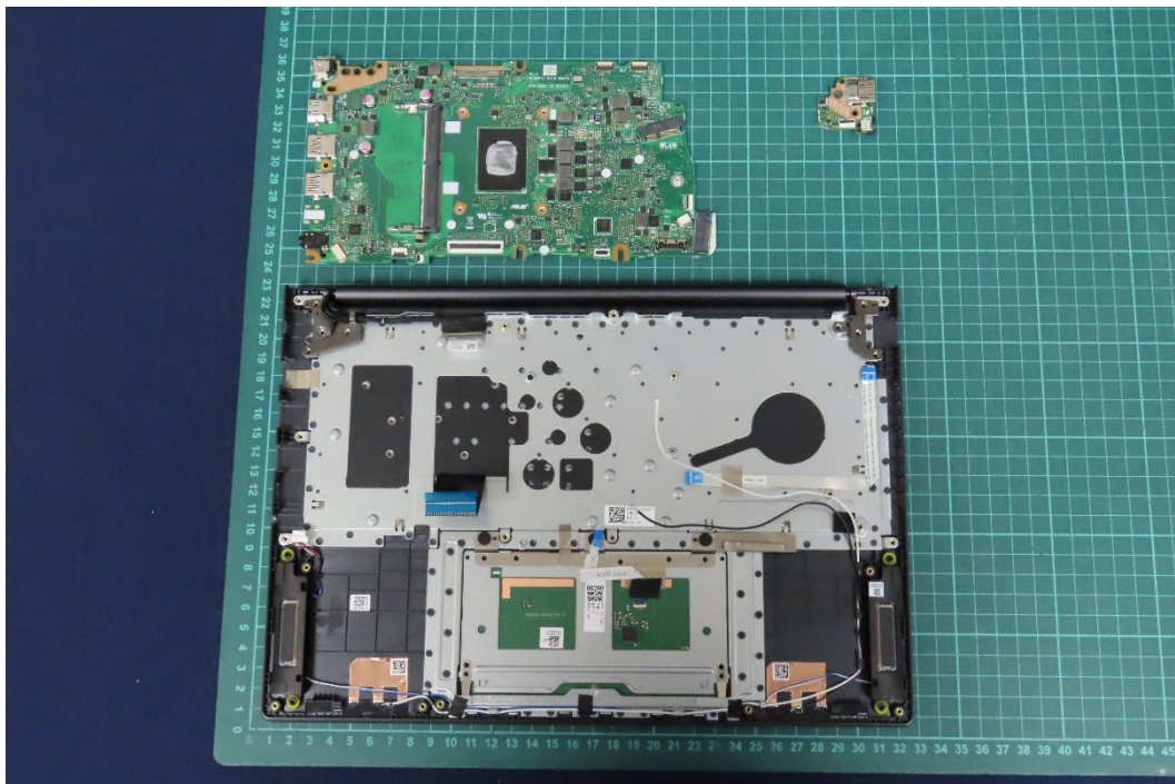
(19) EUT Photo
