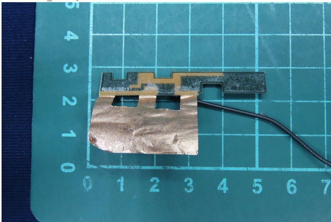
(28) EUT Photo_INPAQ Main Antenna
