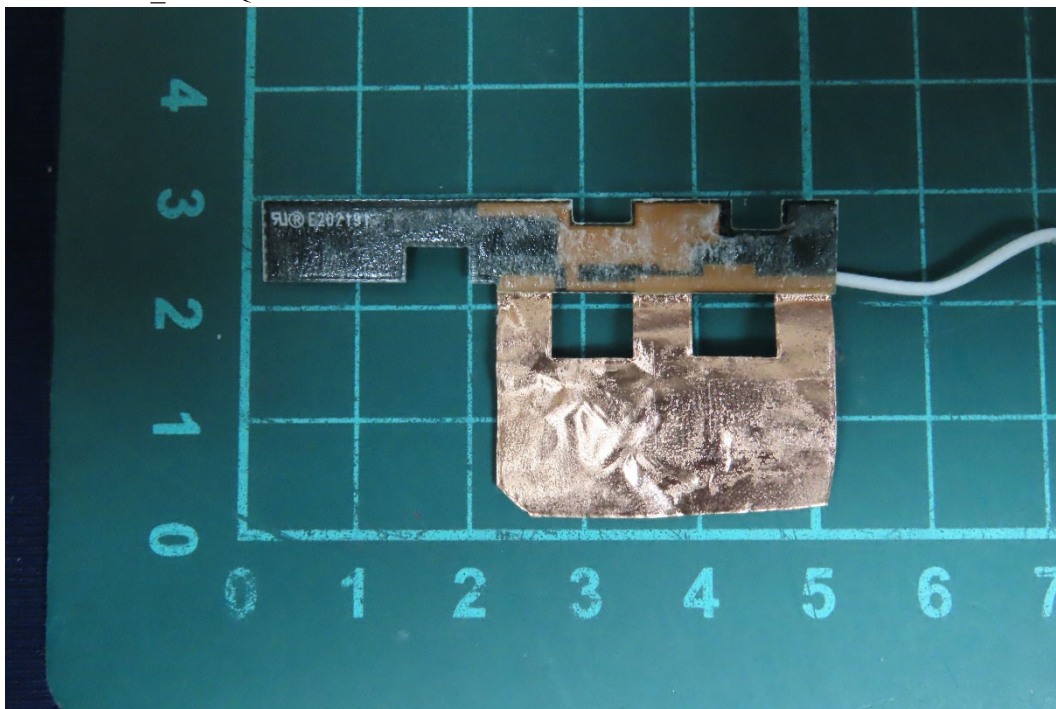
(30) EUT Photo_INPAQ Aux Antenna
