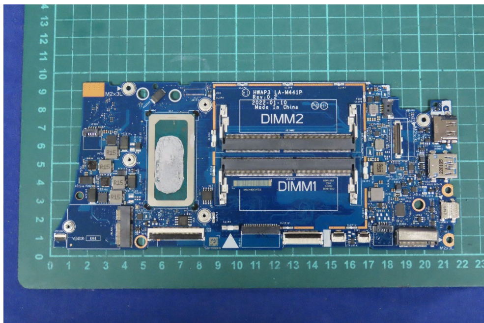
(24) EUT Photo
