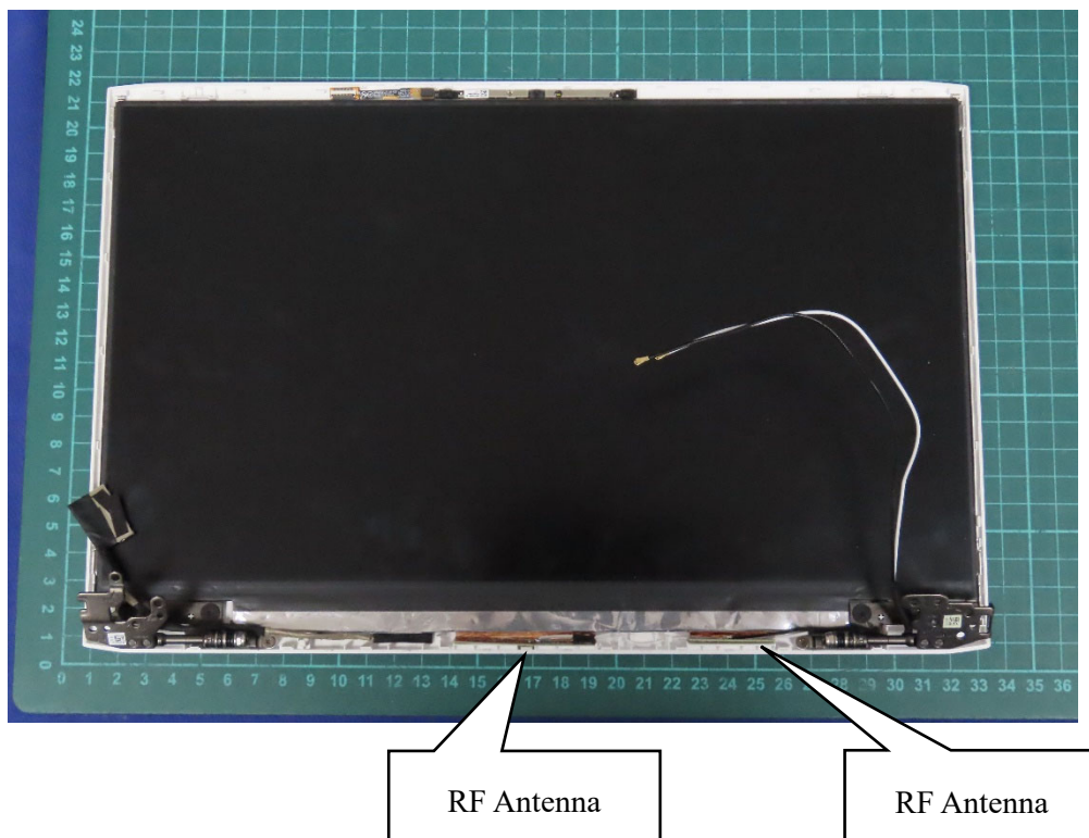
(30) EUT Photo
