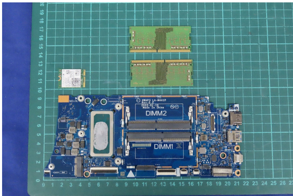
(21) EUT Photo
