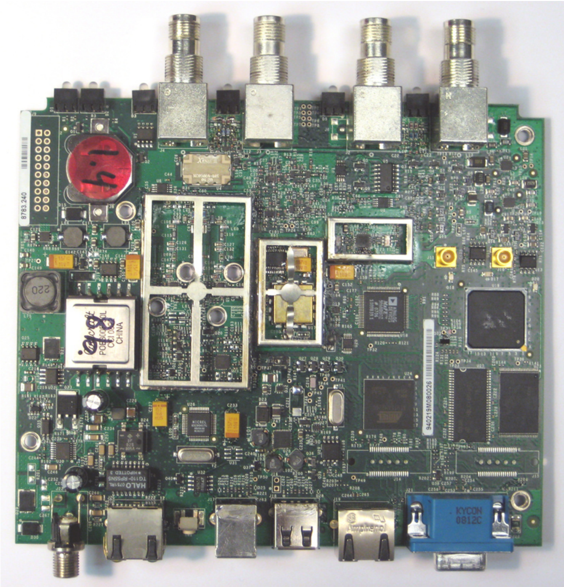
PCB Top
