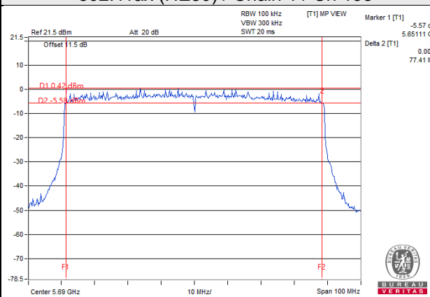
802.11ax (HE80) / Chain 1 / Ch 138
