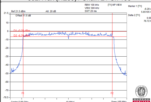
802.11ax (HE80) / Chain 2 / Ch 138
