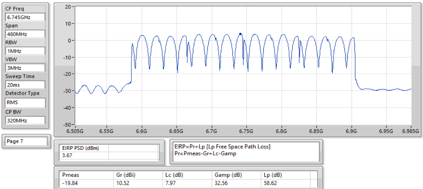
EIRP PSD;Band:6.7G;be320;BWch:320MHz;Nss:1,(M0);Nant:2;Ch:6745MHz;TX
