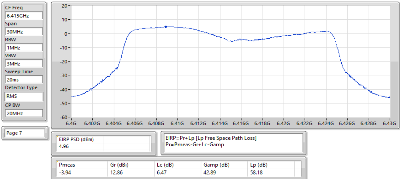
EIRP PSD;Band:6.2G;be20,BF;BWch:20MHz;Nss:1,(M0);Nant:2;Ch:6415MHz;TX
