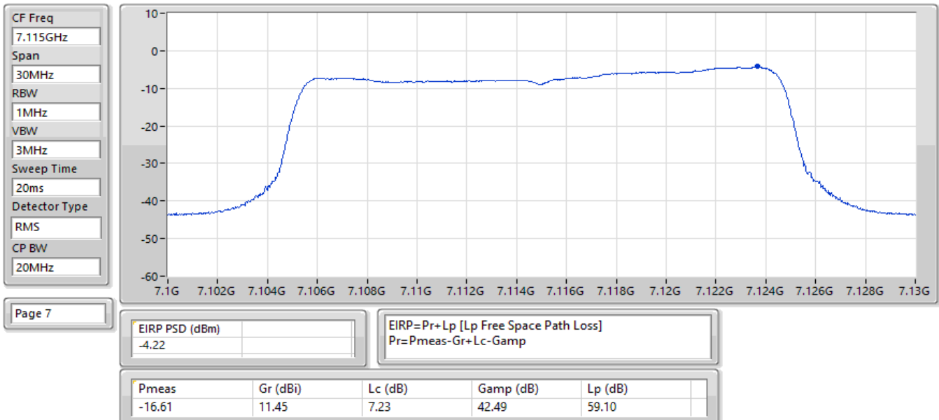
EIRP PSD;Band:7.0G;be20,BF;BWch:20MHz;Nss:1,(M0);Nant:2;Ch:7115MHz;TX
