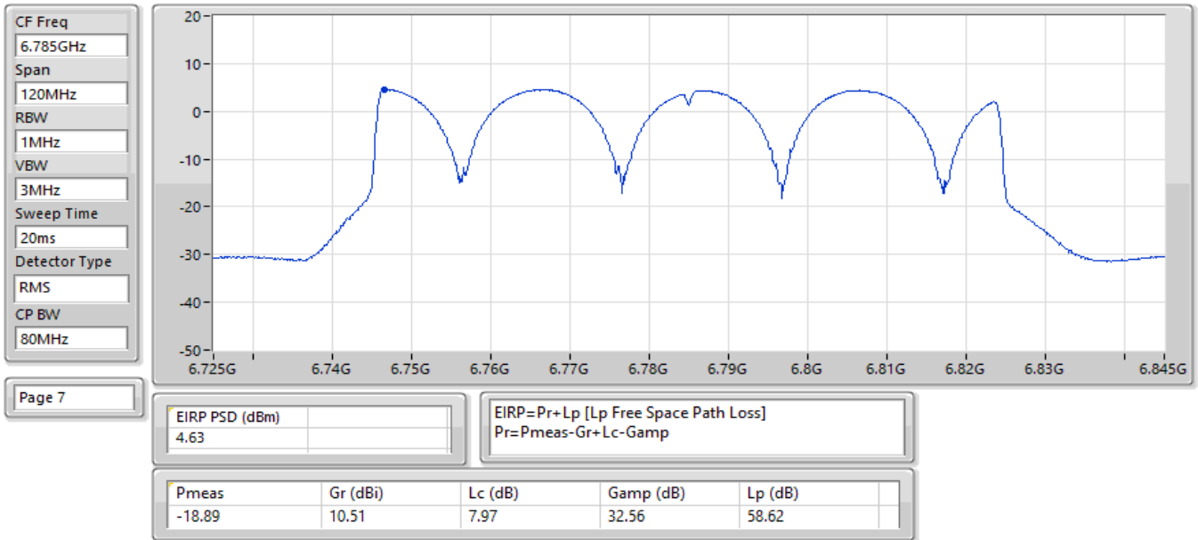
EIRP PSD;Band:6.7G;be80;BWch:80MHz;Nss:1,(M0);Nant:2;Ch:6785MHz;TX
