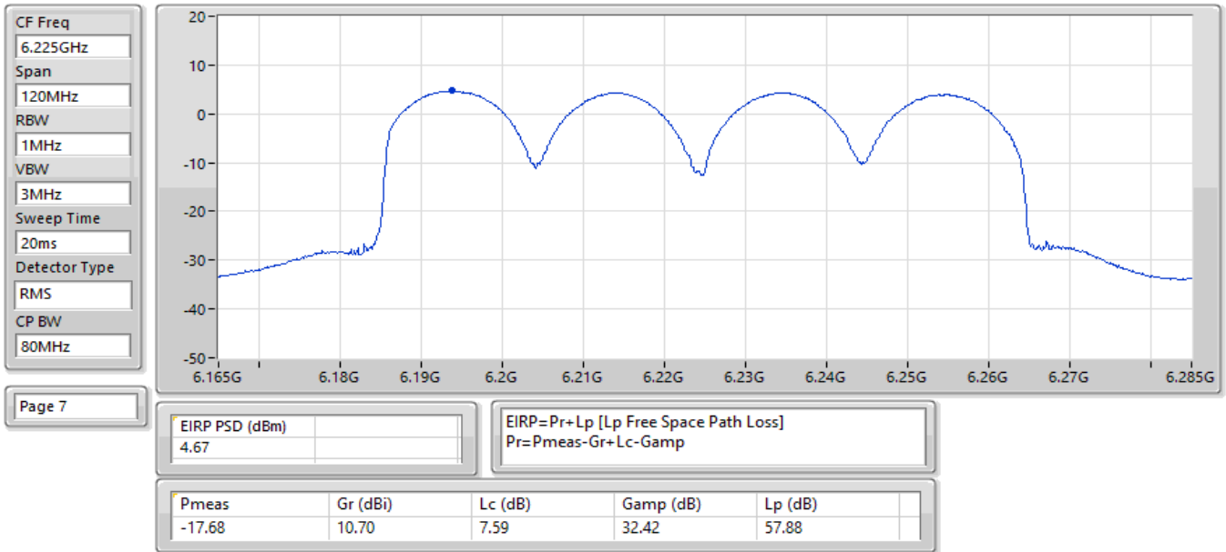
EIRP PSD;Band:6.2G;be80;BWch:80MHz;Nss:1,(M0);Nant:2;Ch:6225MHz;TX
