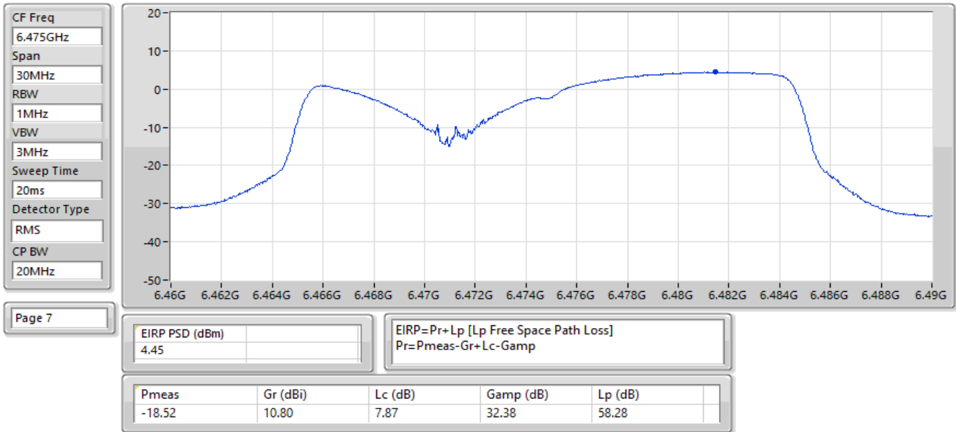
EIRP PSD;Band:6.4G;be20;BWch:20MHz;Nss:1,(M0);Nant:2;Ch:6475MHz;TX
