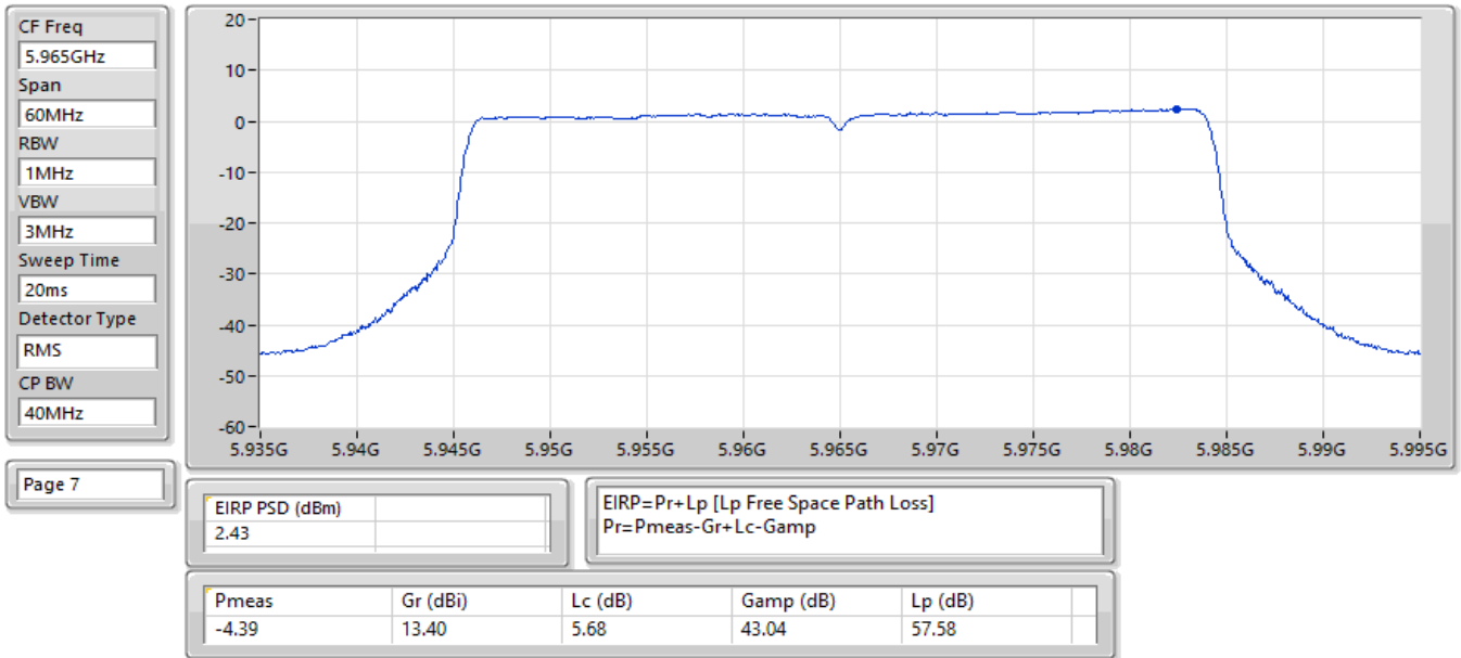
EIRP PSD;Band:6.2G;be40,BF;BWch:40MHz;Nss:1,(M0);Nant:2;Ch:5965MHz;TX
