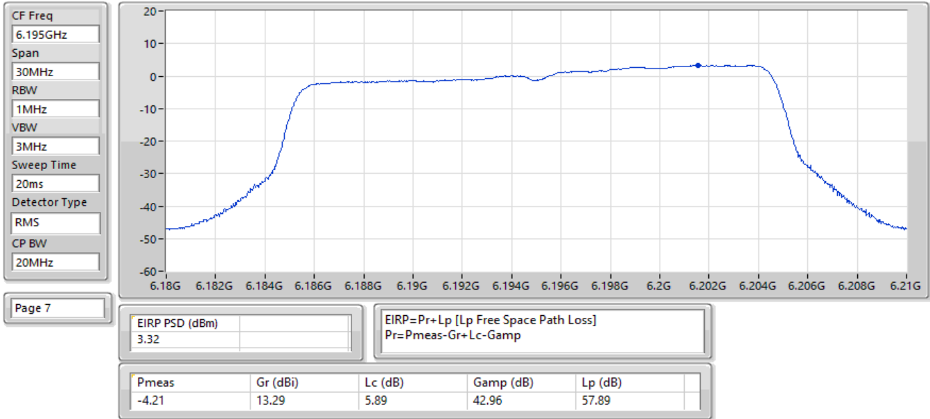
EIRP PSD;Band:6.2G;be20,BF;BWch:20MHz;Nss:1,(M0);Nant:2;Ch:6195MHz;TX
