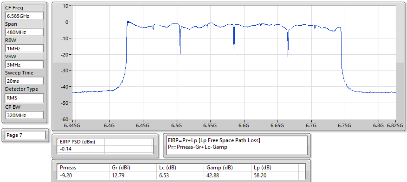
EIRP PSD;Band:6.4G;be320,BF;BWch:320MHz;Nss:1,(M0);Nant:2;Ch:6585MHz;TX
