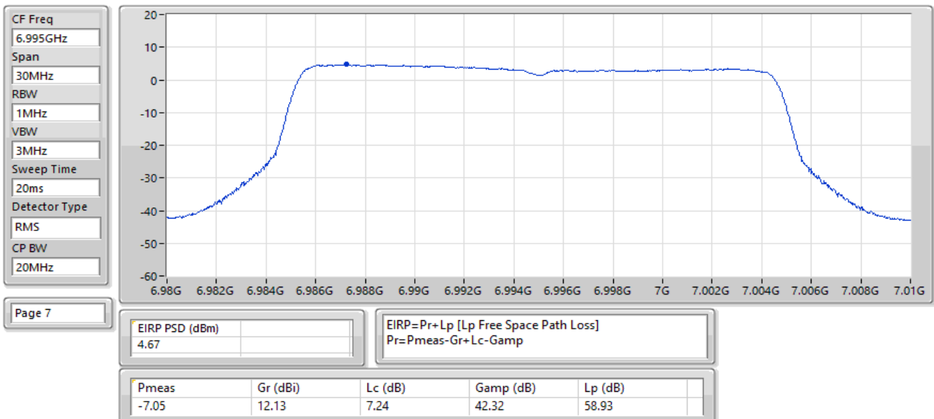
EIRP PSD;Band:7.0G;be20,BF;BWch:20MHz;Nss:1,(M0);Nant:2;Ch:6995MHz;TX
