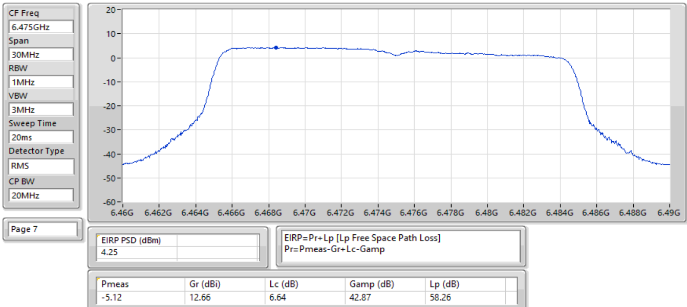
EIRP PSD;Band:6.4G;be20,BF;BWch:20MHz;Nss:1,(M0);Nant:2;Ch:6475MHz;TX
