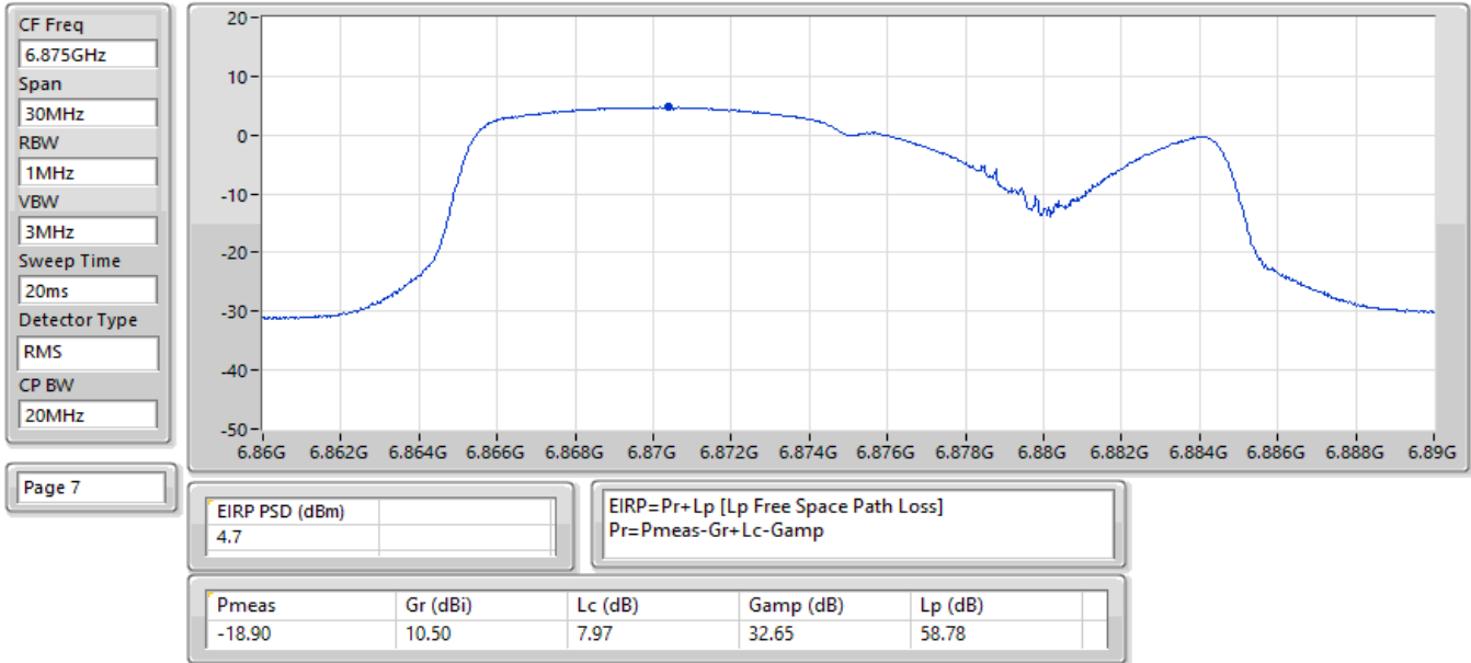
EIRP PSD;Band:6.7G;be20;BWch:20MHz;Nss:1,(M0);Nant:2;Ch:6875MHz;TX
