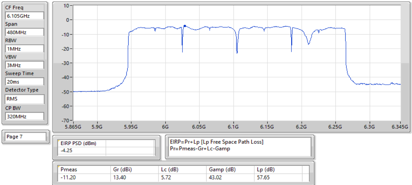
EIRP PSD;Band:6.2G;be320,BF;BWch:320MHz;Nss:1,(M0);Nant:2;Ch:6105MHz;TX
