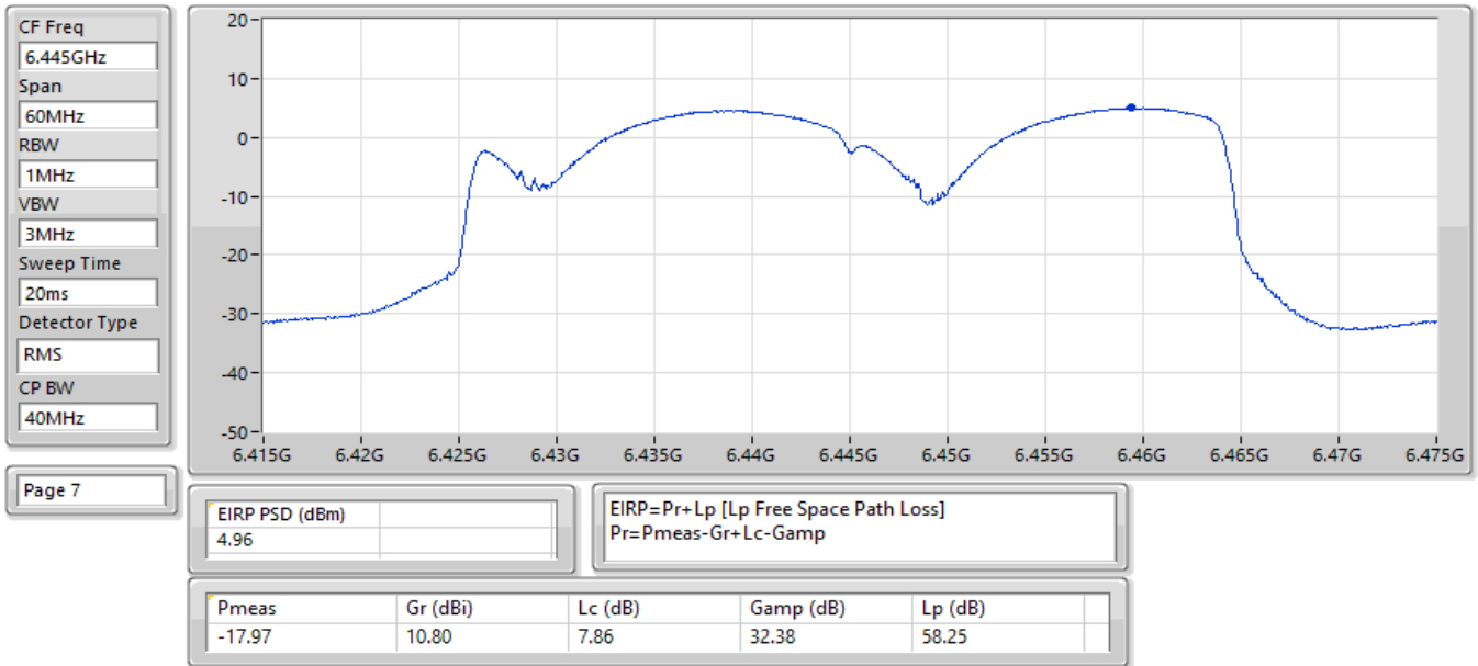
EIRP PSD;Band:6.4G;be40;BWch:40MHz;Nss:1,(M0);Nant:2;Ch:6445MHz;TX
