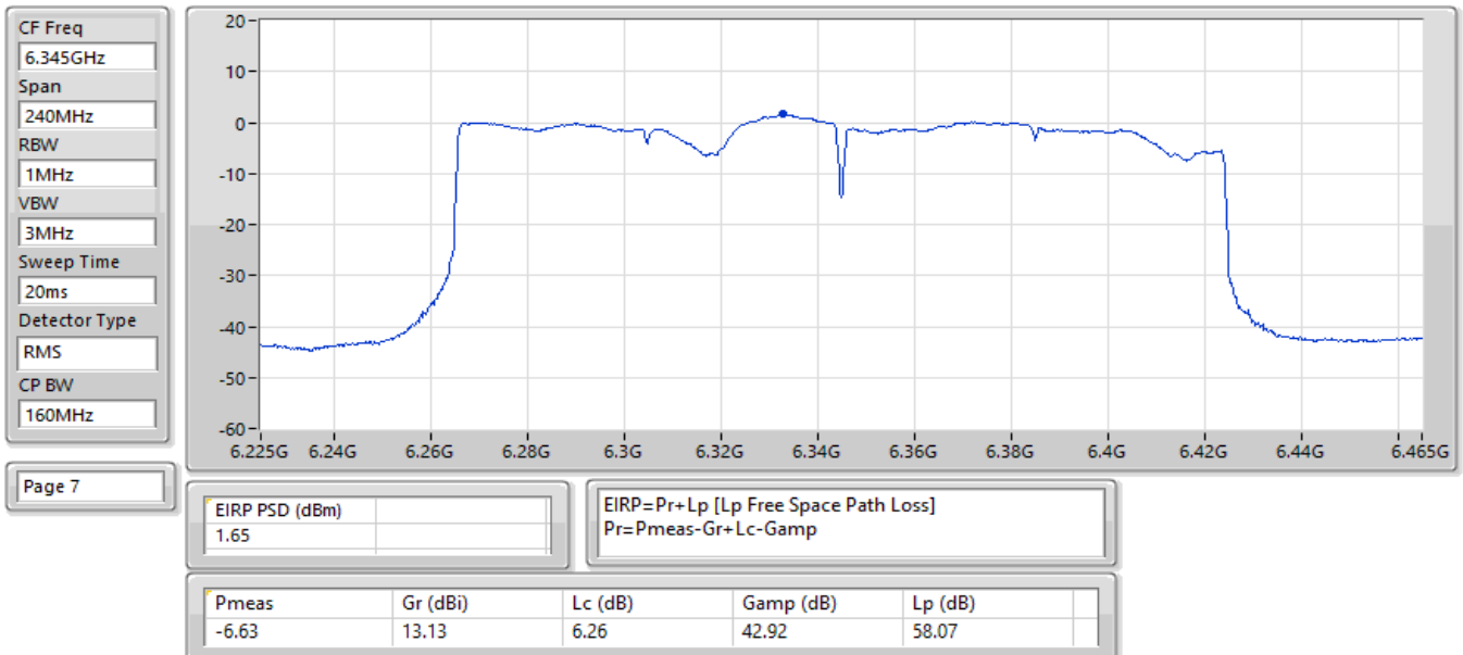
EIRP PSD;Band:6.2G;be160,BF;BWch:160MHz;Nss:1,(M0);Nant:2;Ch:6345MHz;TX
