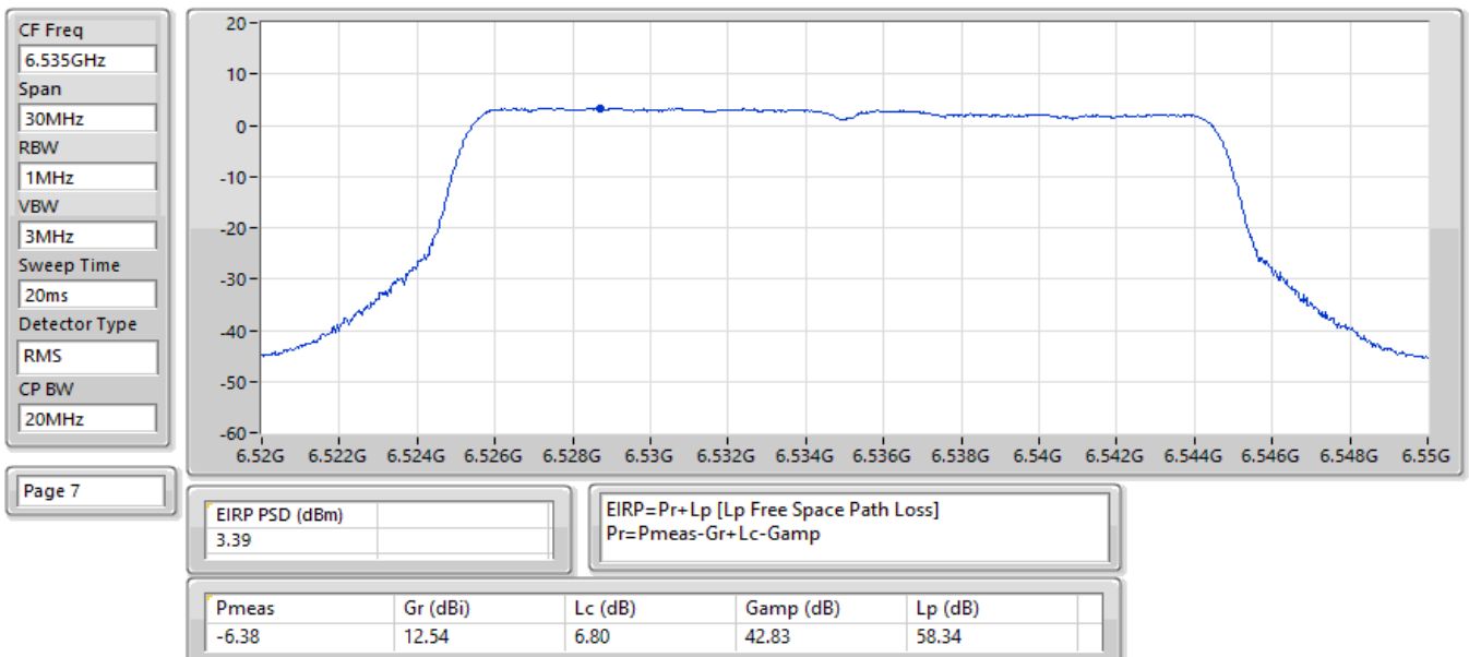
EIRP PSD;Band:6.7G;be20,BF;BWch:20MHz;Nss:1,(M0);Nant:2;Ch:6535MHz;TX
