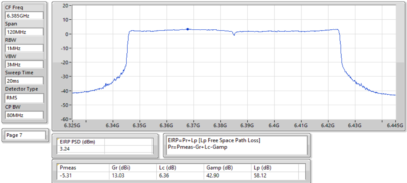
EIRP PSD;Band:6.2G;be80,BF;BWch:80MHz;Nss:1,(M0);Nant:2;Ch:6385MHz;TX
