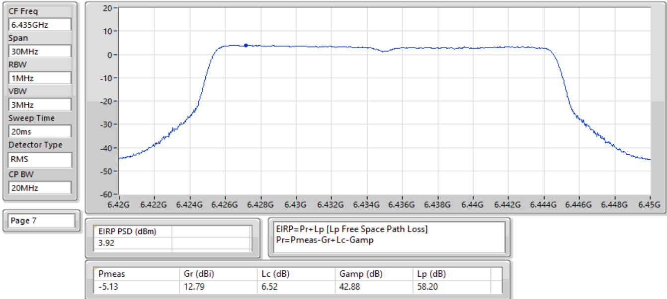
EIRP PSD;Band:6.4G;be20,BF;BWch:20MHz;Nss:1,(M0);Nant:2;Ch:6435MHz;TX
