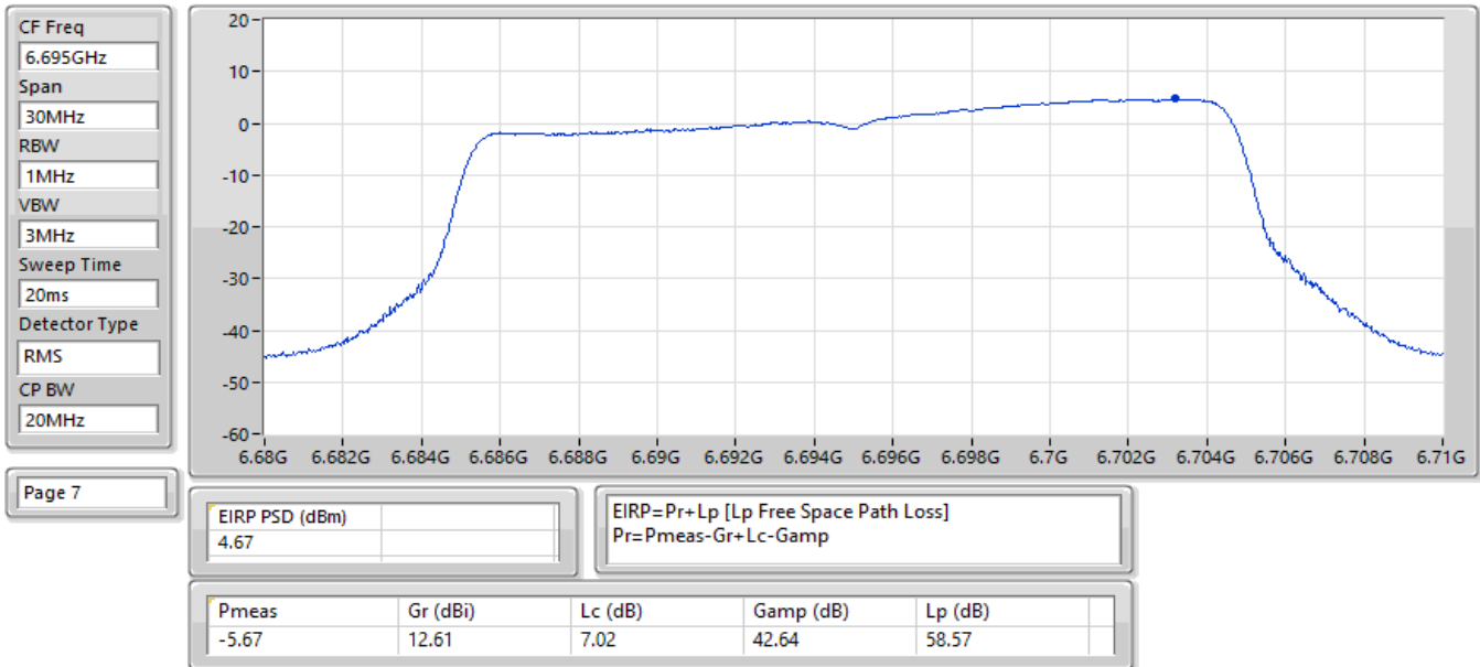
EIRP PSD;Band:6.7G;be20,BF;BWch:20MHz;Nss:1,(M0);Nant:2;Ch:6695MHz;TX
