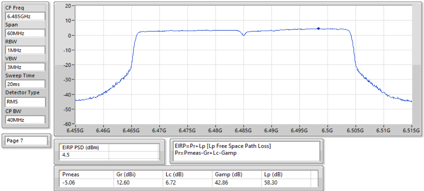
EIRP PSD;Band:6.4G;be40,BF;BWch:40MHz;Nss:1,(M0);Nant:2;Ch:6485MHz;TX
