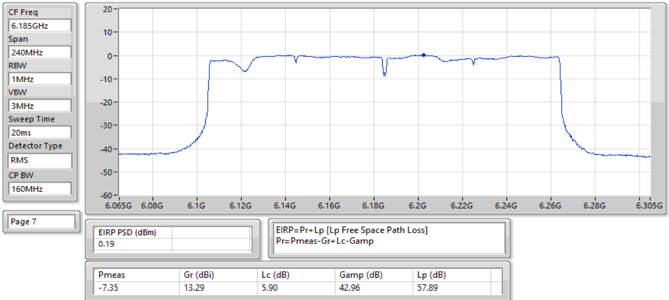
EIRP PSD;Band:6.2G;be160,BF;BWch:160MHz;Nss:1,(M0);Nant:2;Ch:6185MHz;TX
