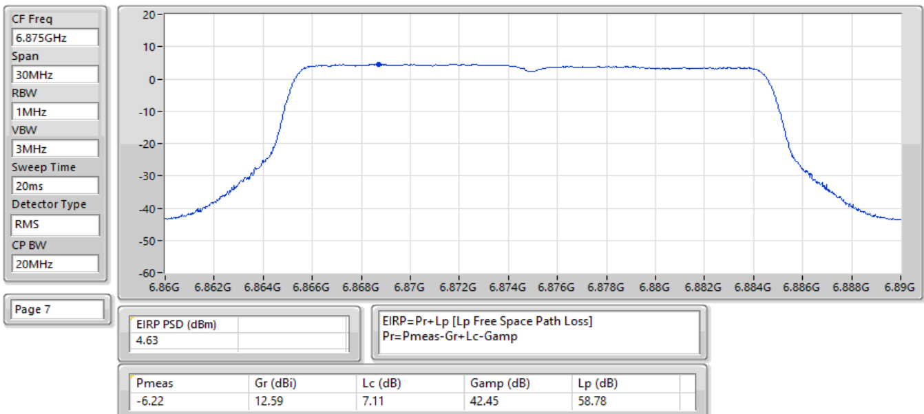
EIRP PSD;Band:6.7G;be20,BF;BWch:20MHz;Nss:1,(M0);Nant:2;Ch:6875MHz;TX
