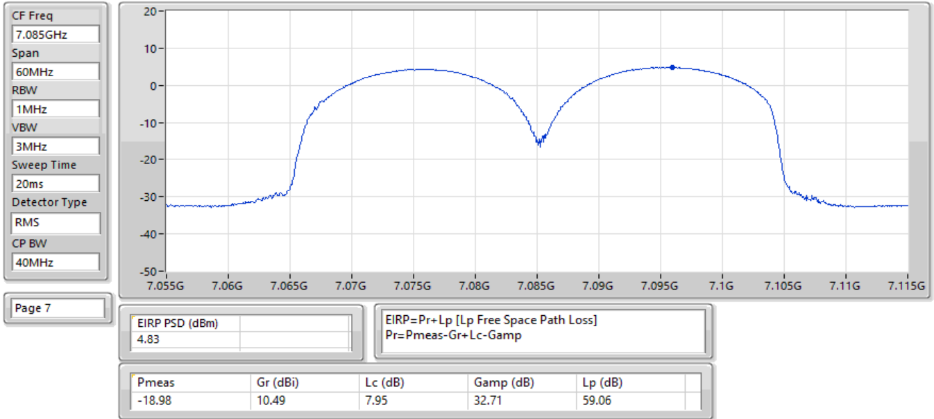
EIRP PSD;Band:7.0G;be40;BWch:40MHz;Nss:1,(M0);Nant:2;Ch:7085MHz;TX
