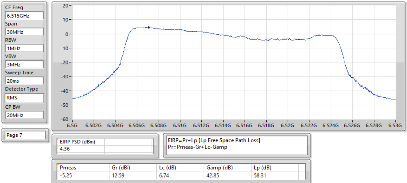
EIRP PSD;Band:6.4G;be20,BF;BWch:20MHz;Nss:1,(M0);Nant:2;Ch:6515MHz;TX
