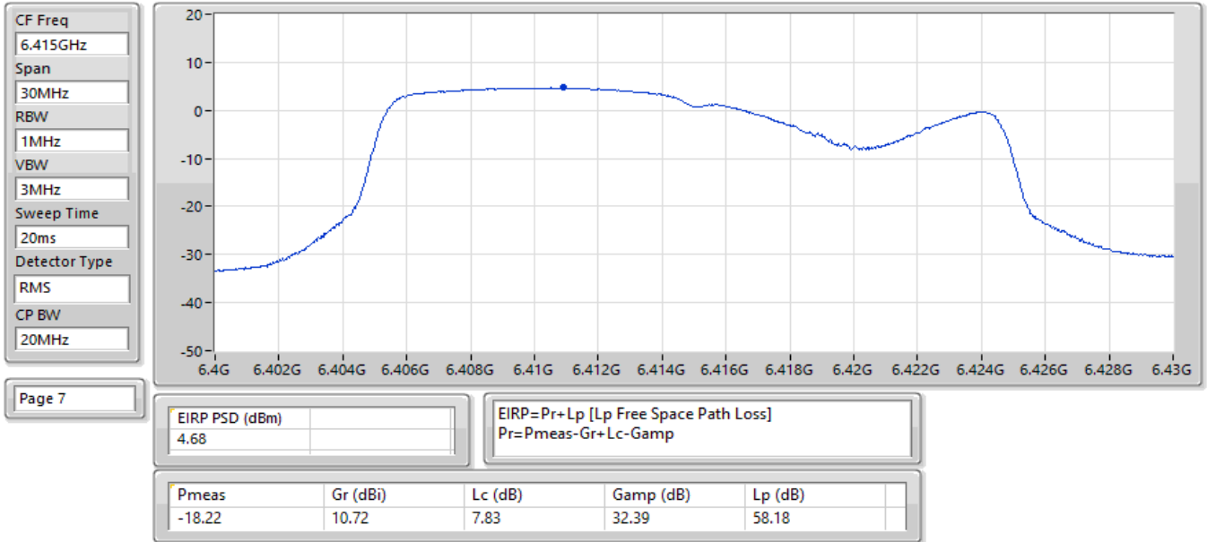
EIRP PSD;Band:6.2G;be20;BWch:20MHz;Nss:1,(M0);Nant:2;Ch:6415MHz;TX
