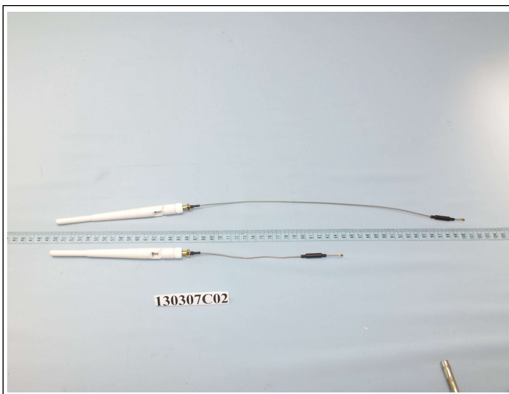
Set 5 antenna
