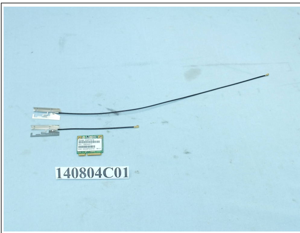
Set 1 antenna
