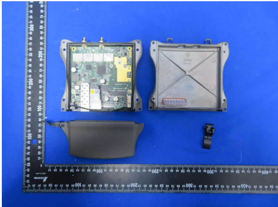
(2) EUT Photo
