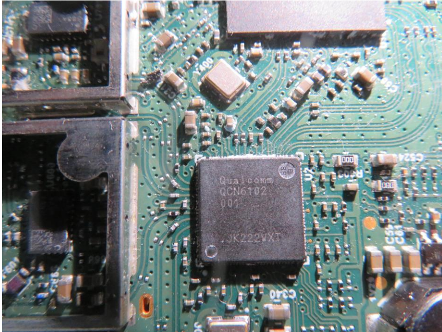
(9) EUT Photo
