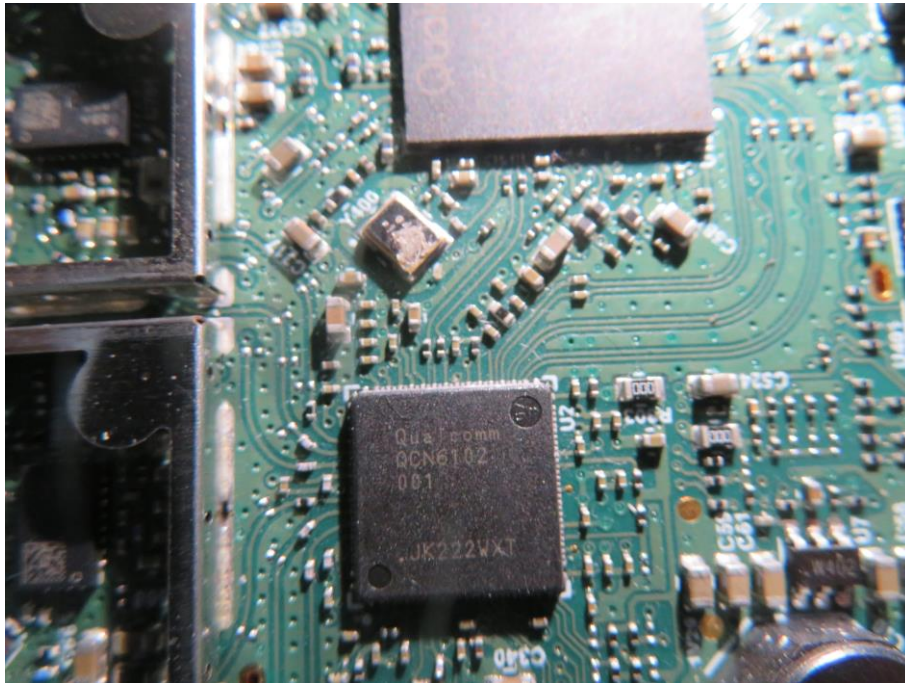
(5) EUT Photo
