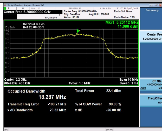
11AX20MIMO-Ant2-5200
