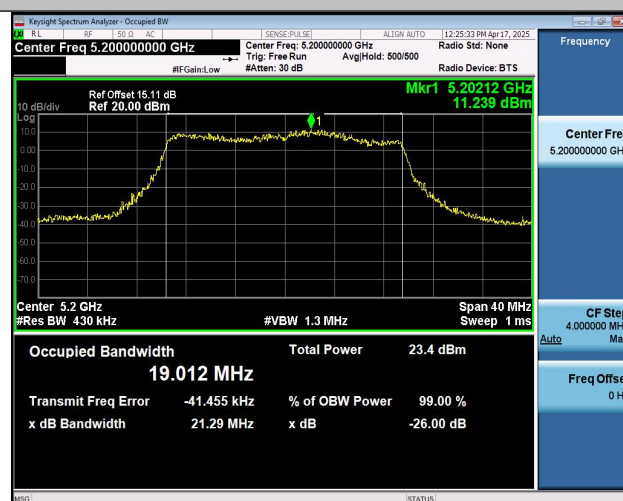
11AX20MIMO-Ant3-5200
