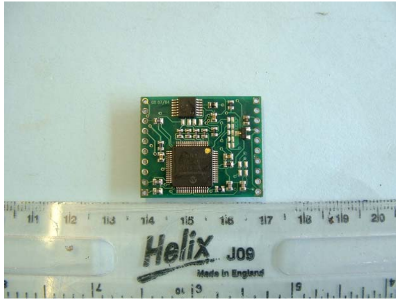
RF Module Bottom Side
