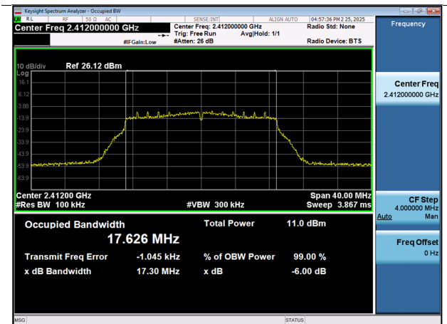
802.11n_HT20-CH 1
