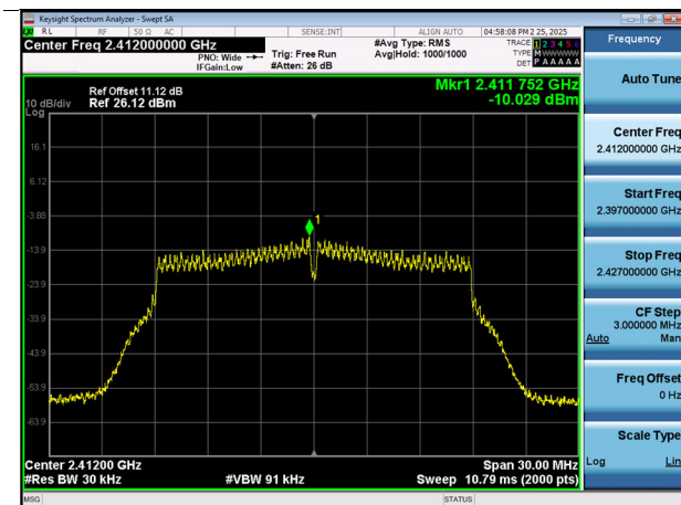
802.11n_HT20-CH 1
