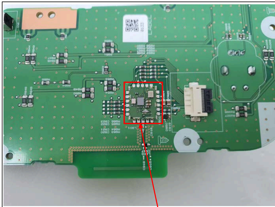
BT Module
