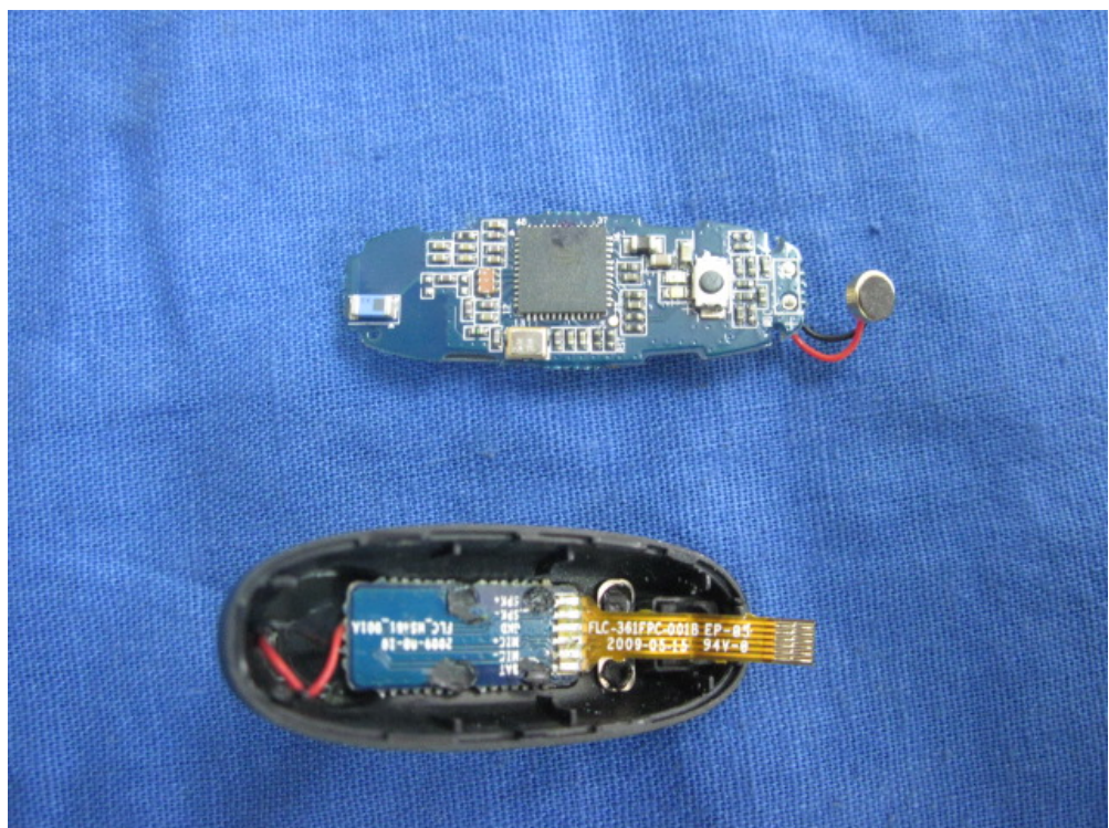
(13) EUT Photo
