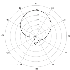
E-Plane HPBW
