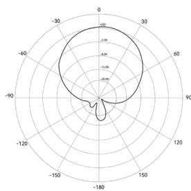
H-Plane HPBW
