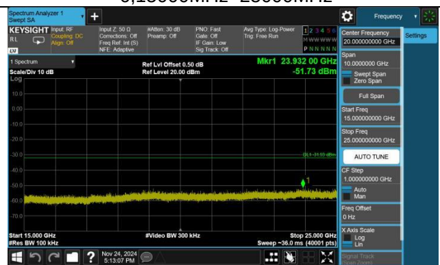
802.11n(HT40),2452MHz,Ant0,Plot 6,15000MHz~25000MHz
