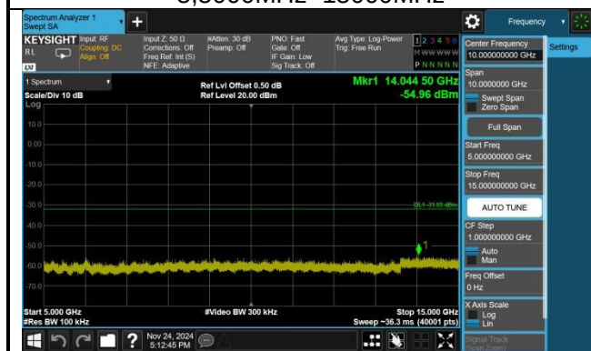
802.11n(HT40),2452MHz,Ant0,Plot 5,5000MHz~15000MHz
