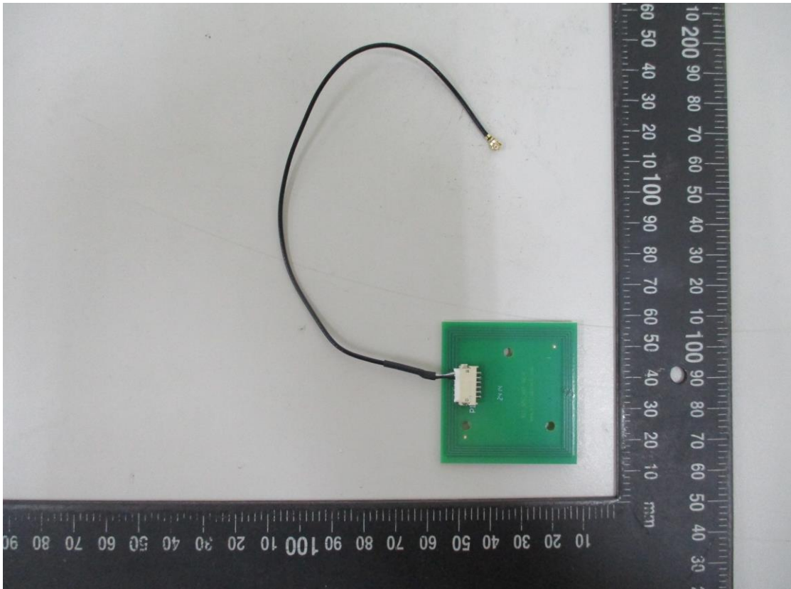
RFID Antenna
