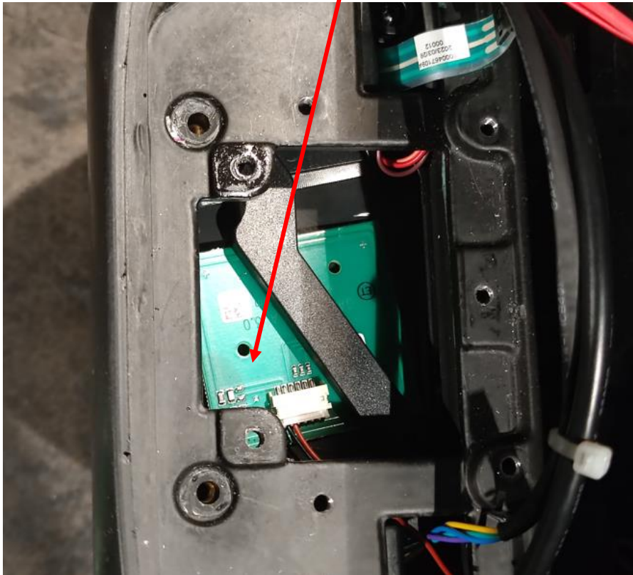
RFID Antenna
