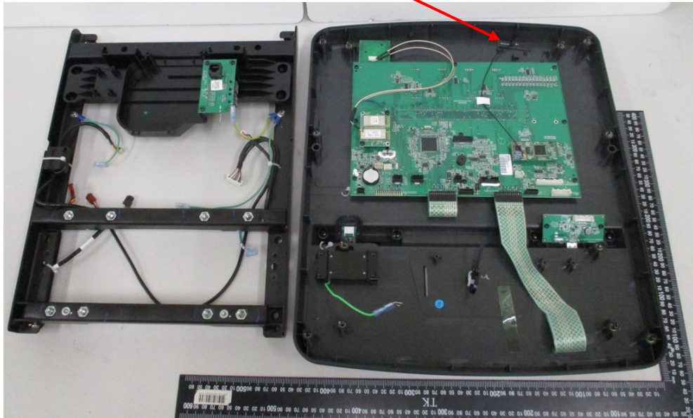
Antenna
