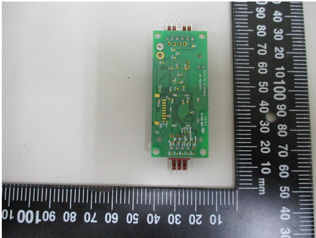
RFID module
