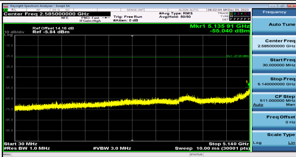
11N20MIMO-Ant0-5240-30~5140
