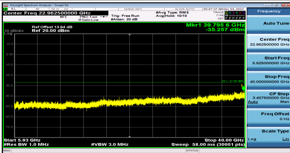
11A-Ant0-5745-5925~40000
