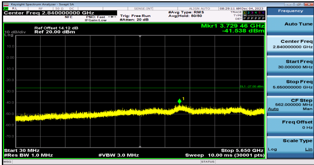
11N20MIMO-Ant1-5745-30~5650
