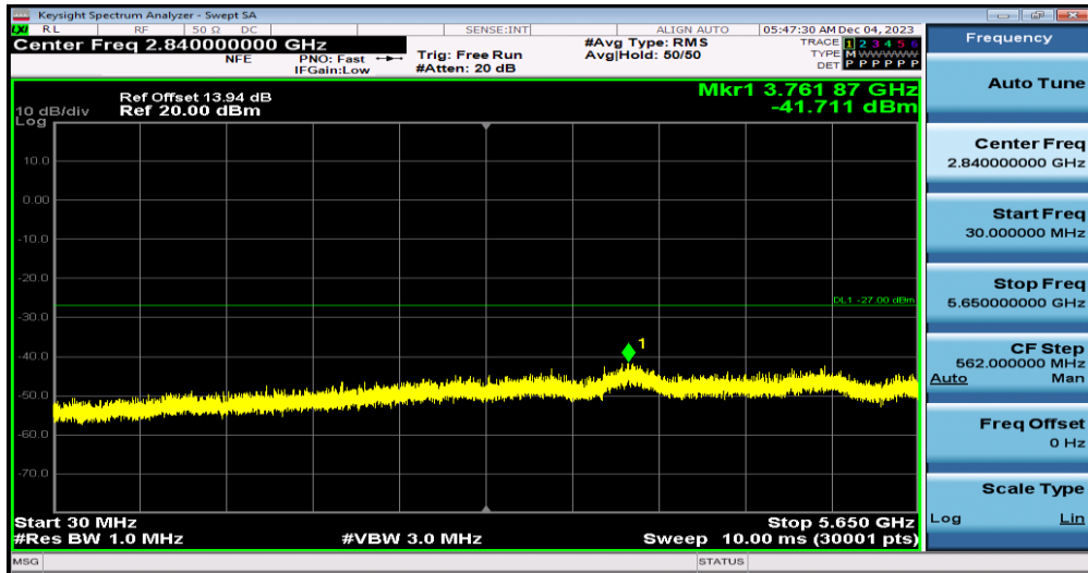
11A-Ant0-5745-30~5650
