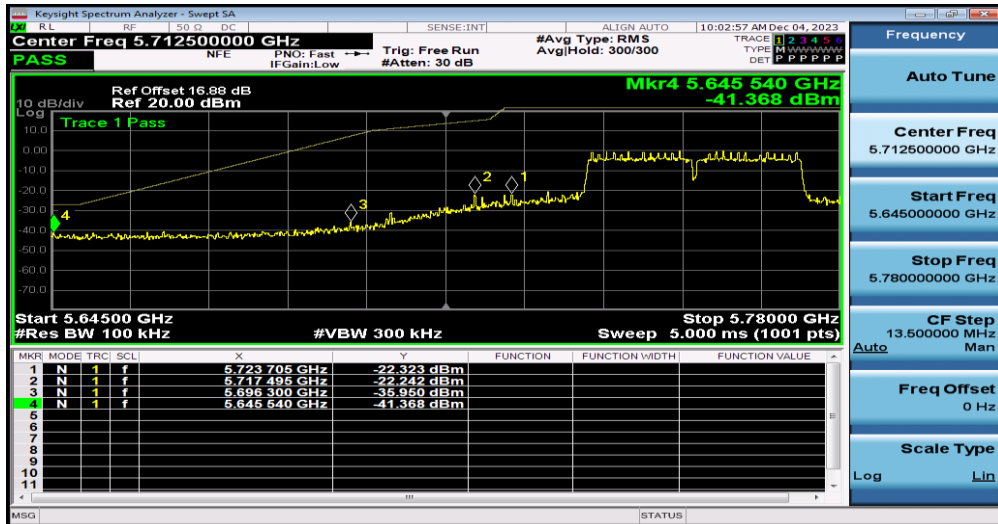
11N40MIMO-Ant1-5755
