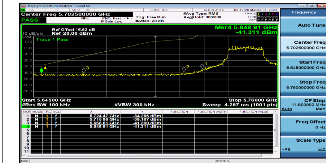
11A-Ant1-5745
