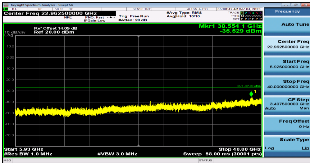
11A-Ant0-5825-5925~40000
