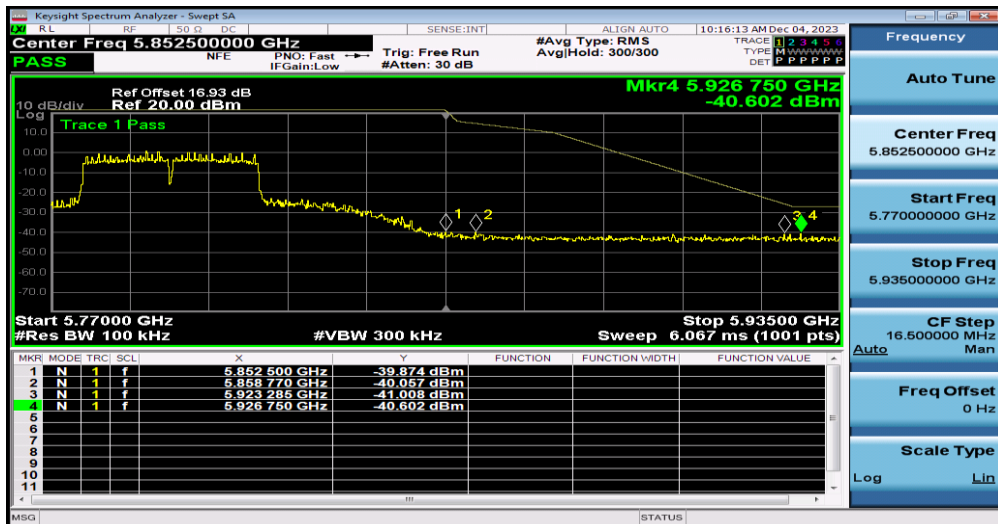
11N40MIMO-Ant0-5795
