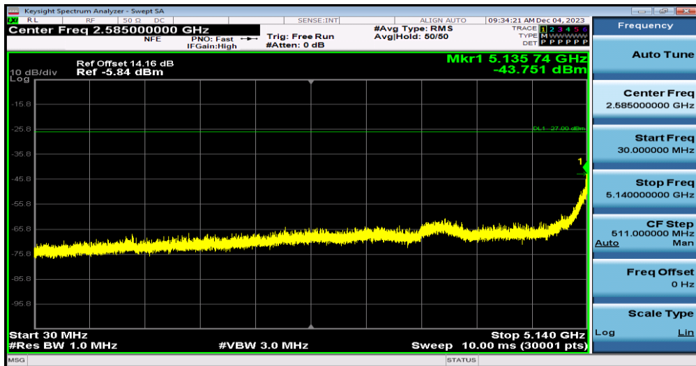
11N40MIMO-Ant0-5230-30~5140
