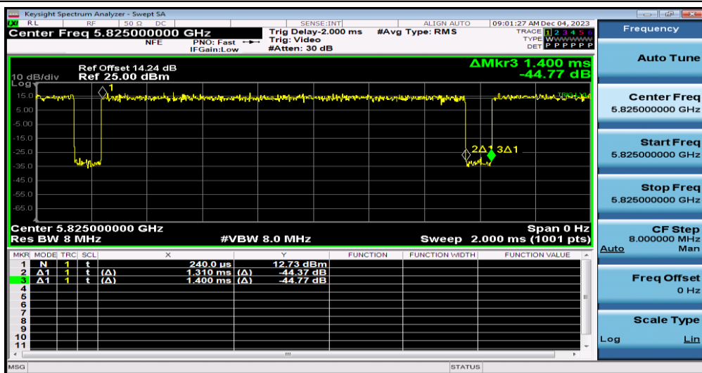
NTNV-11N20MIMO-Ant1-5825
