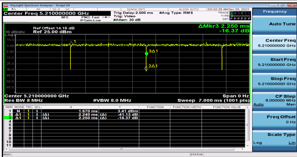
NTNV-11AC80MIMO-Ant0-5210
