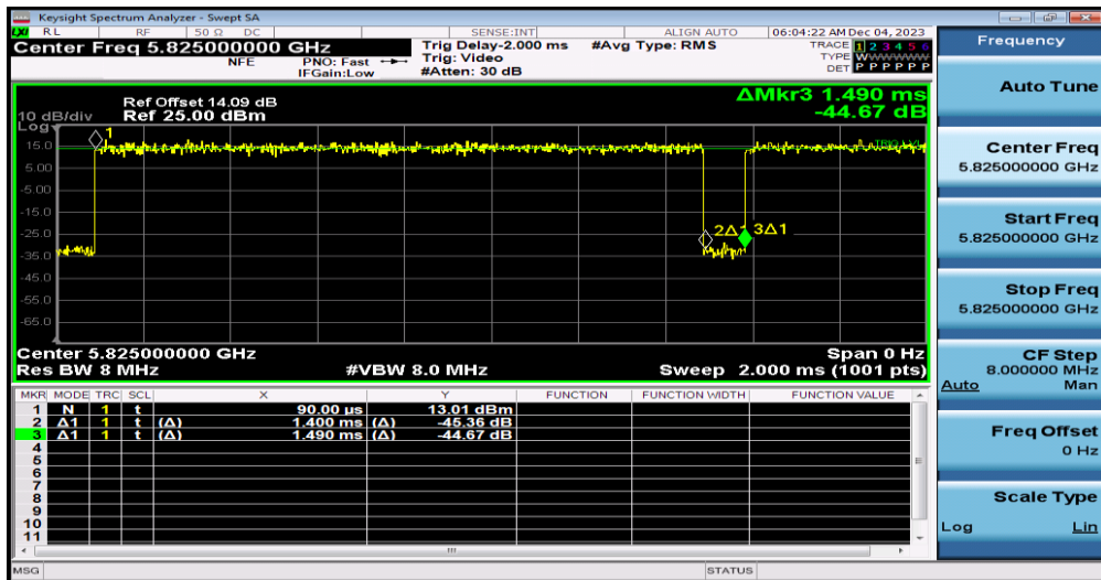
NTNV-11A-Ant0-5825
