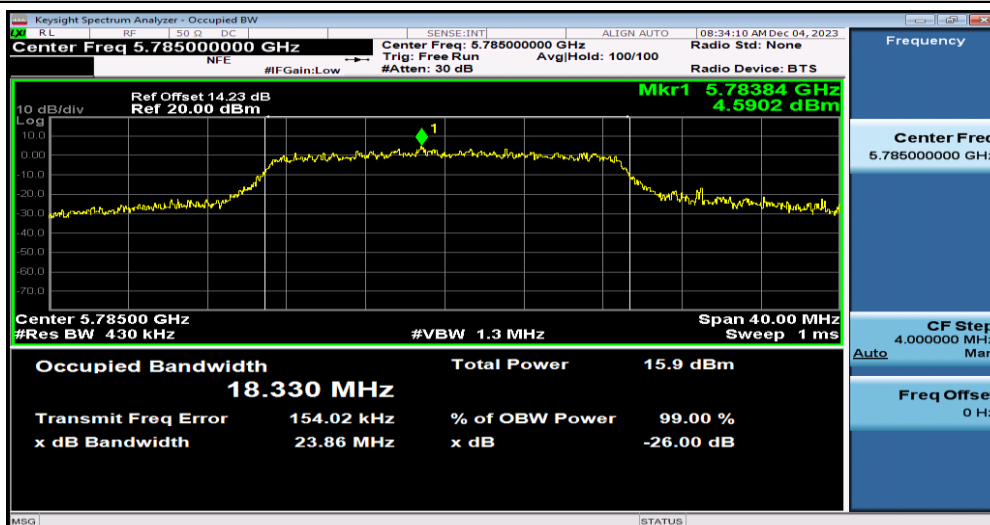
11N20MIMO-Ant0-5785
