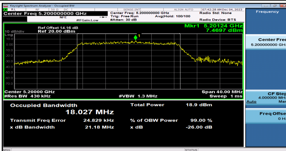
11N20MIMO-Ant0-5200
