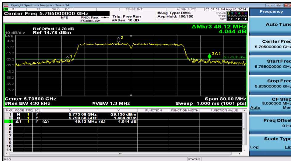
11N40MIMO-Ant1-5795
