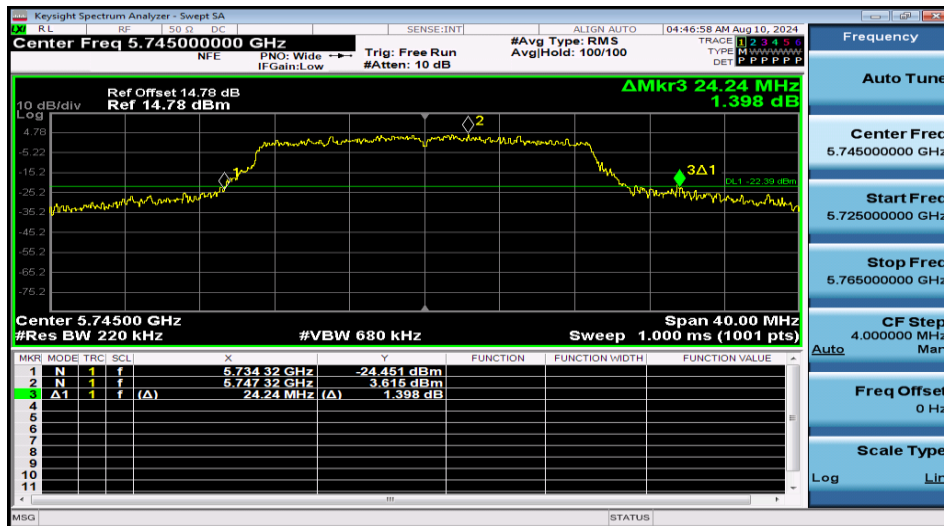
11N20MIMO-Ant1-5745
