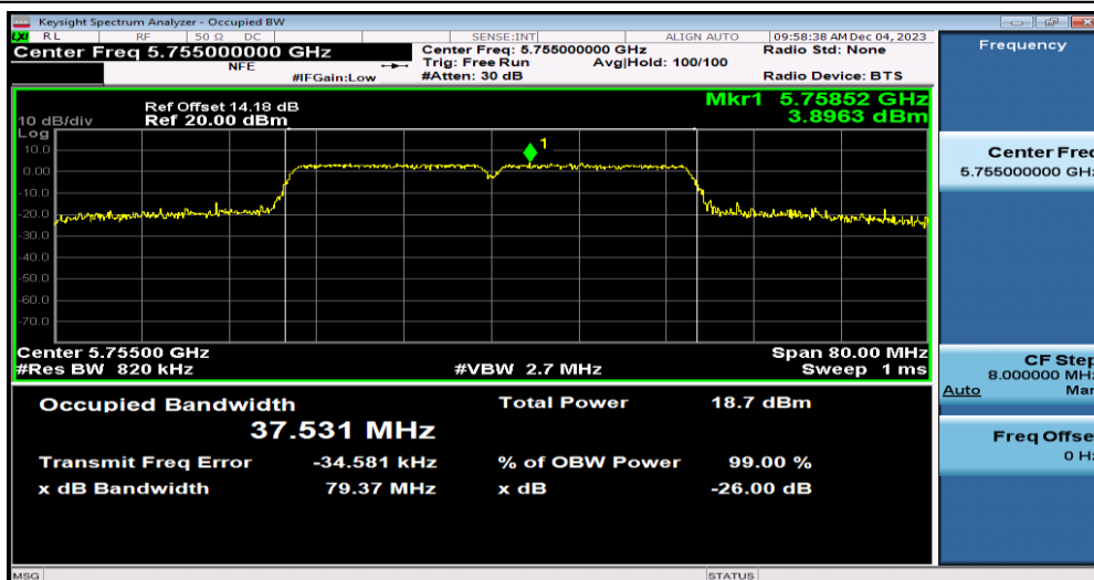
11N40MIMO-Ant1-5755
