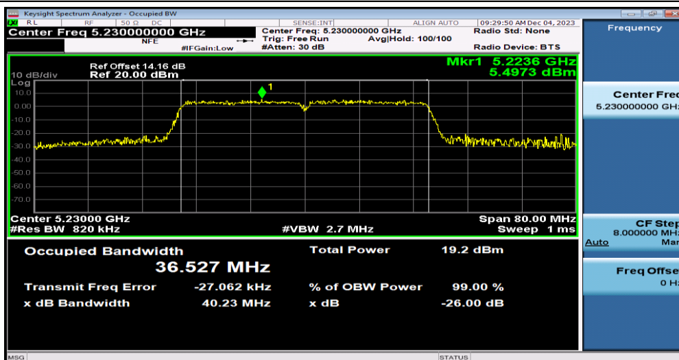
11N40MIMO-Ant0-5230
