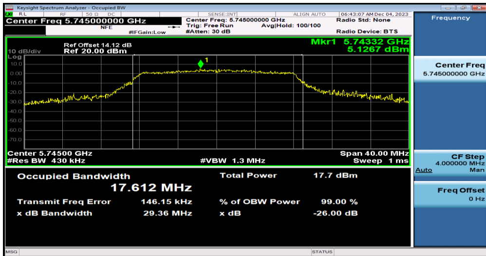
11A-Ant1-5745
