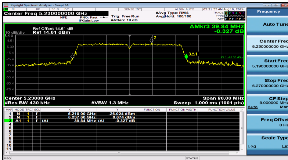
11N40MIMO-Ant1-5230
