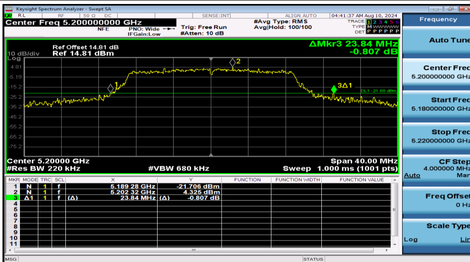
11N20MIMO-Ant1-5200
