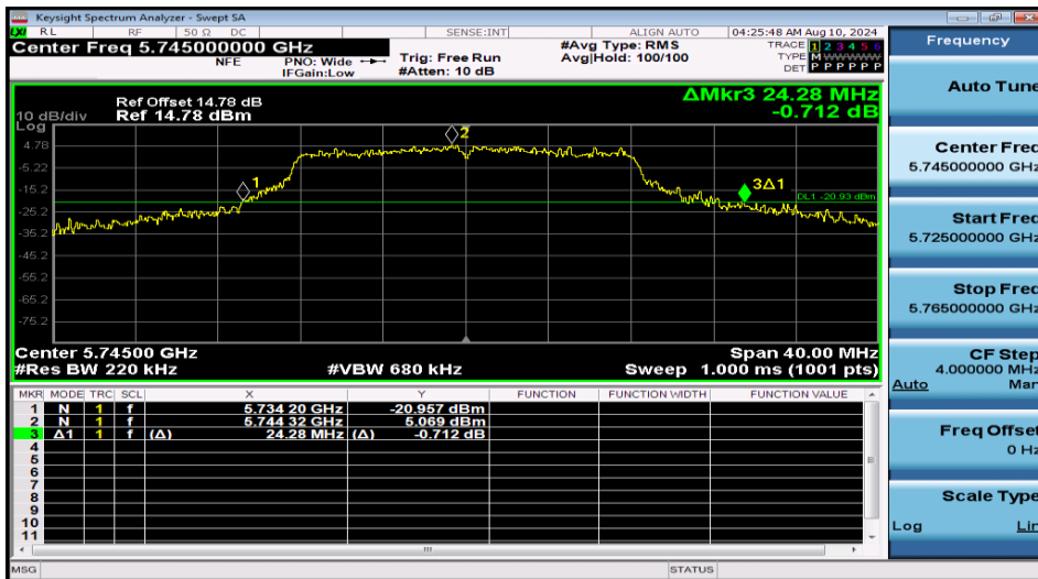
11A-Ant1-5745
