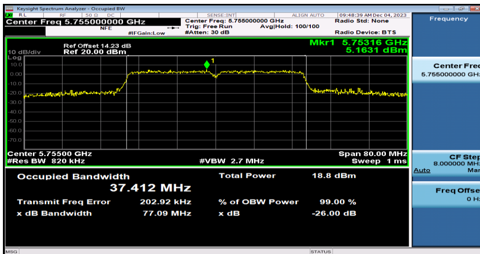
11N40MIMO-Ant0-5755
