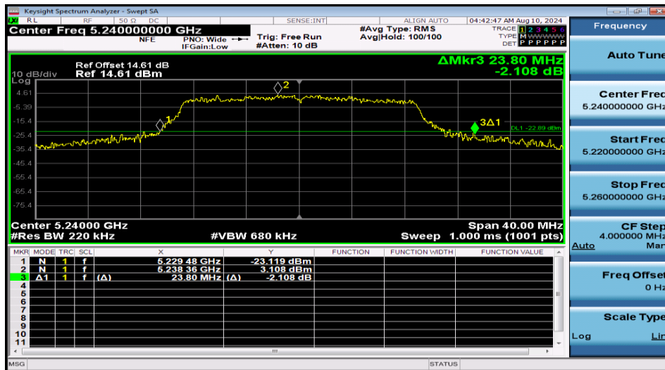
11N20MIMO-Ant1-5240
