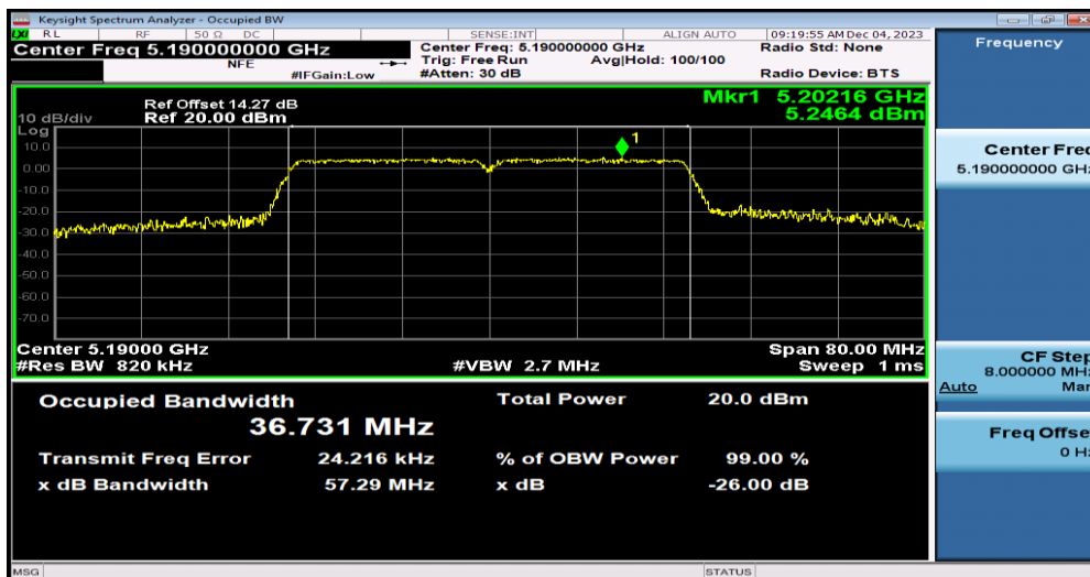
11N40MIMO-Ant1-5190
