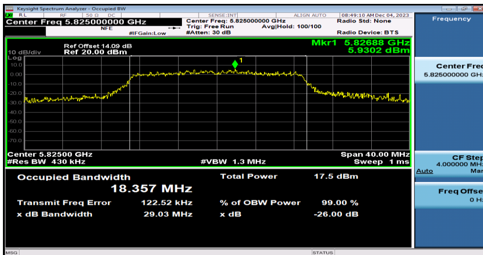
11N20MIMO-Ant0-5825
