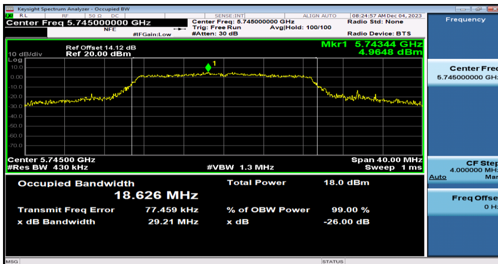
11N20MIMO-Ant1-5745
