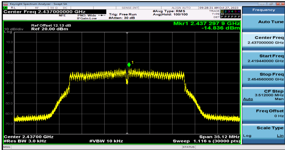
11N20MIMO-Ant1-2437
