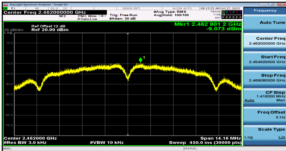
11B-Ant0-2462
