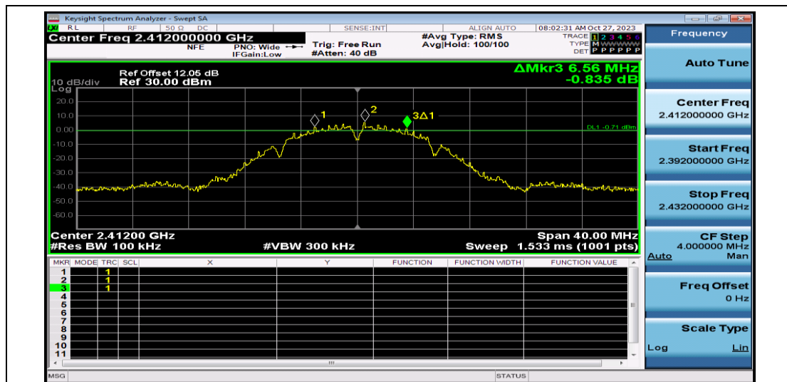
11B-Ant0-2412
