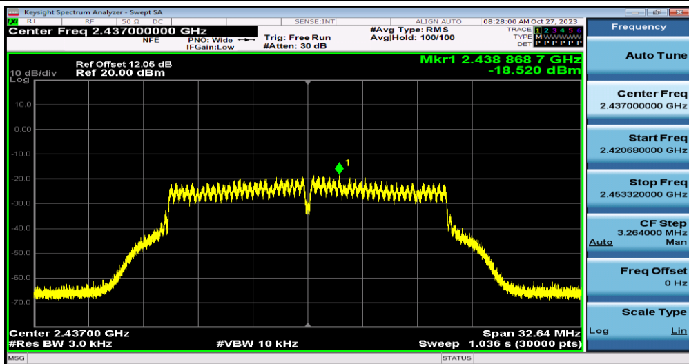
11G-Ant0-2437
