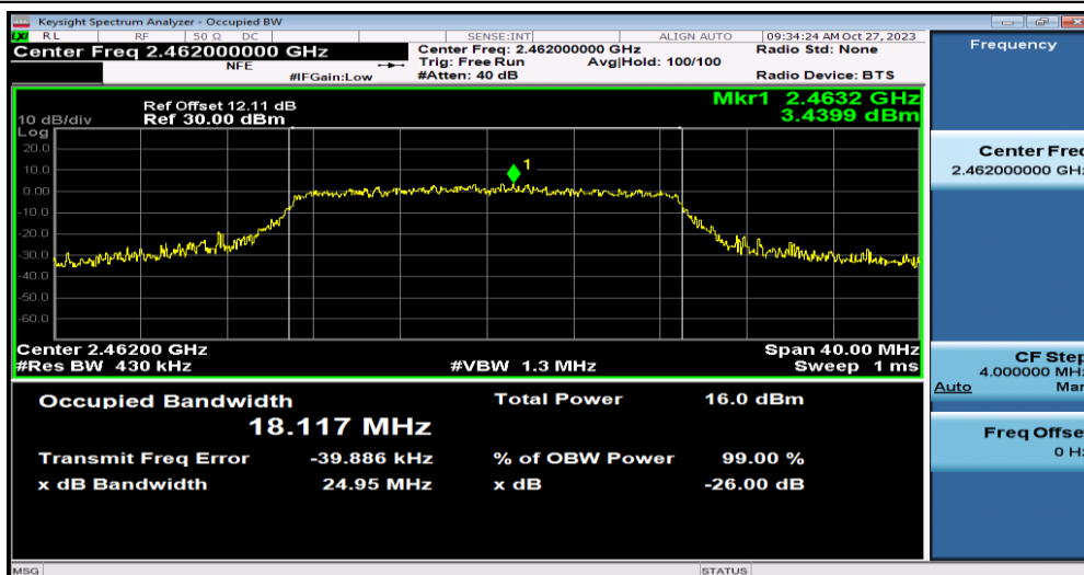
11N20MIMO-Ant1-2462
