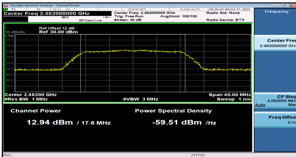
11N20MIMO-Ant0-2462
