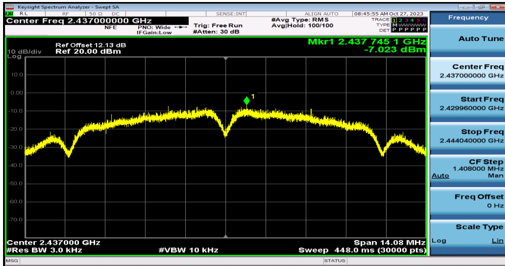
11B-Ant1-2437
