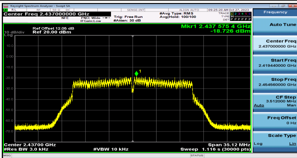
11N20MIMO-Ant0-2437
