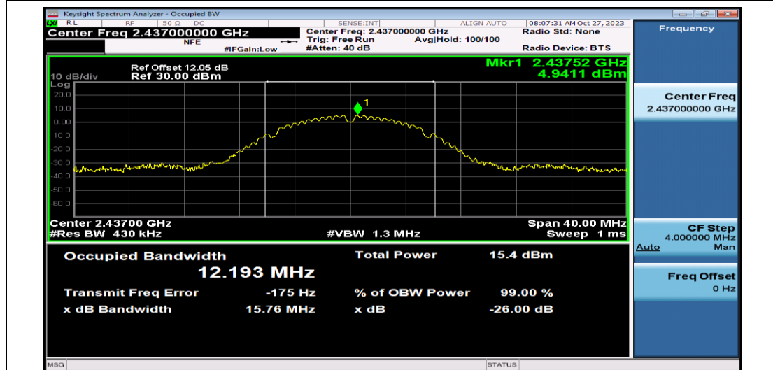
11B-Ant0-2437
