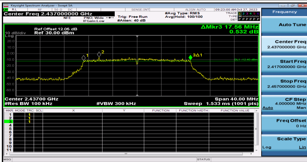
11N20MIMO-Ant0-2437
