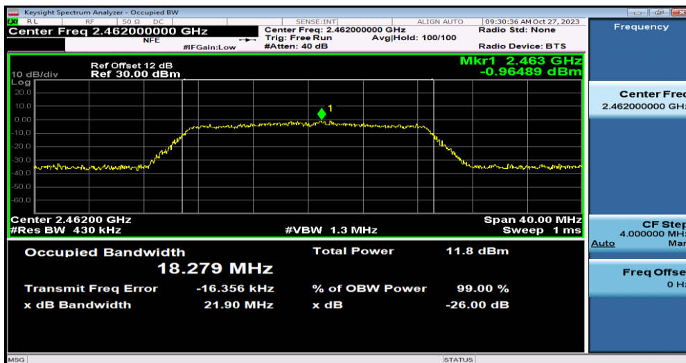
11N20MIMO-Ant0-2462
