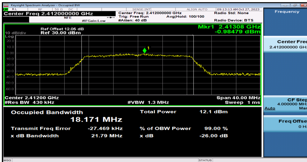
11N20MIMO-Ant0-2412
