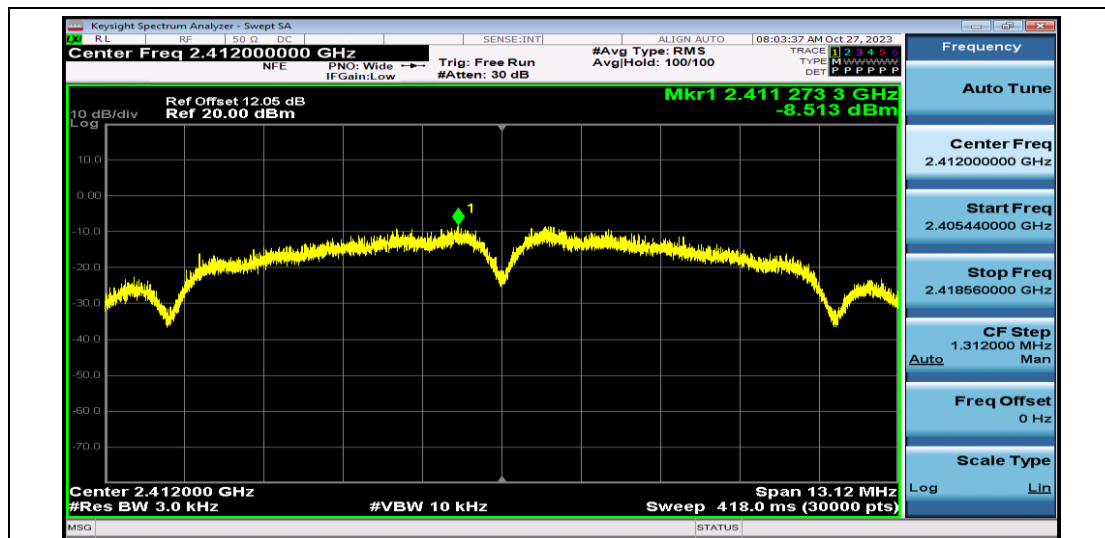
11B-Ant0-2412
