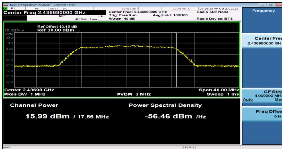
11N20MIMO-Ant1-2437
