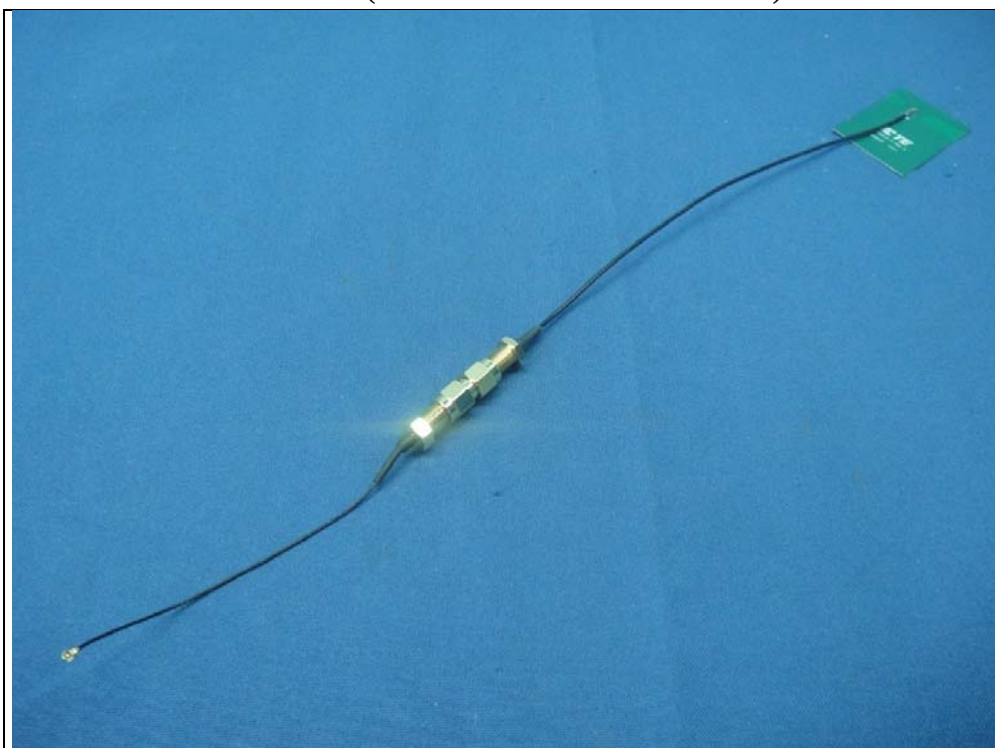
Antenna 1 (Brand: TE / Model: 2118433-1)
