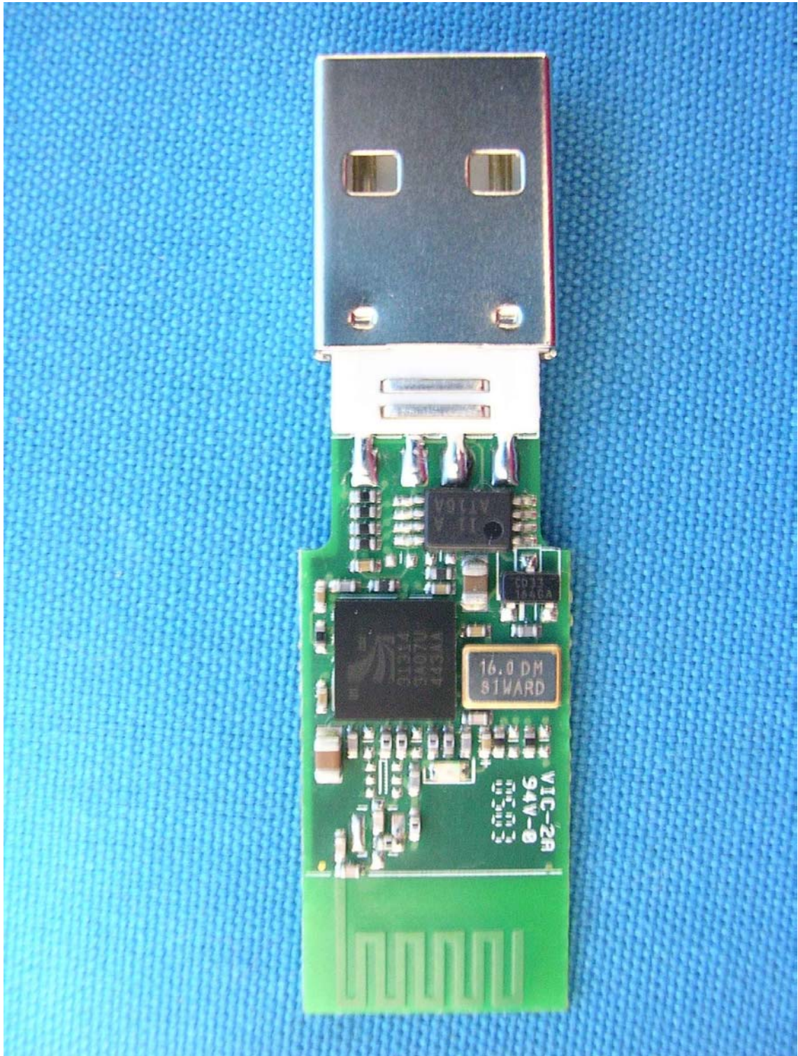
(5) EUT Photo
