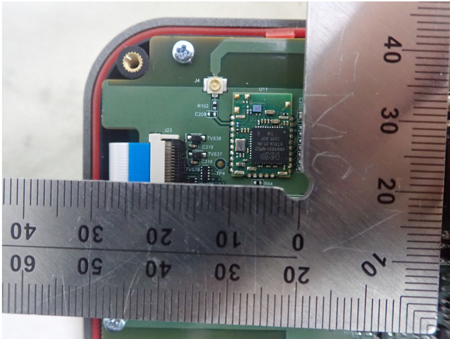
RF Module Front-2
