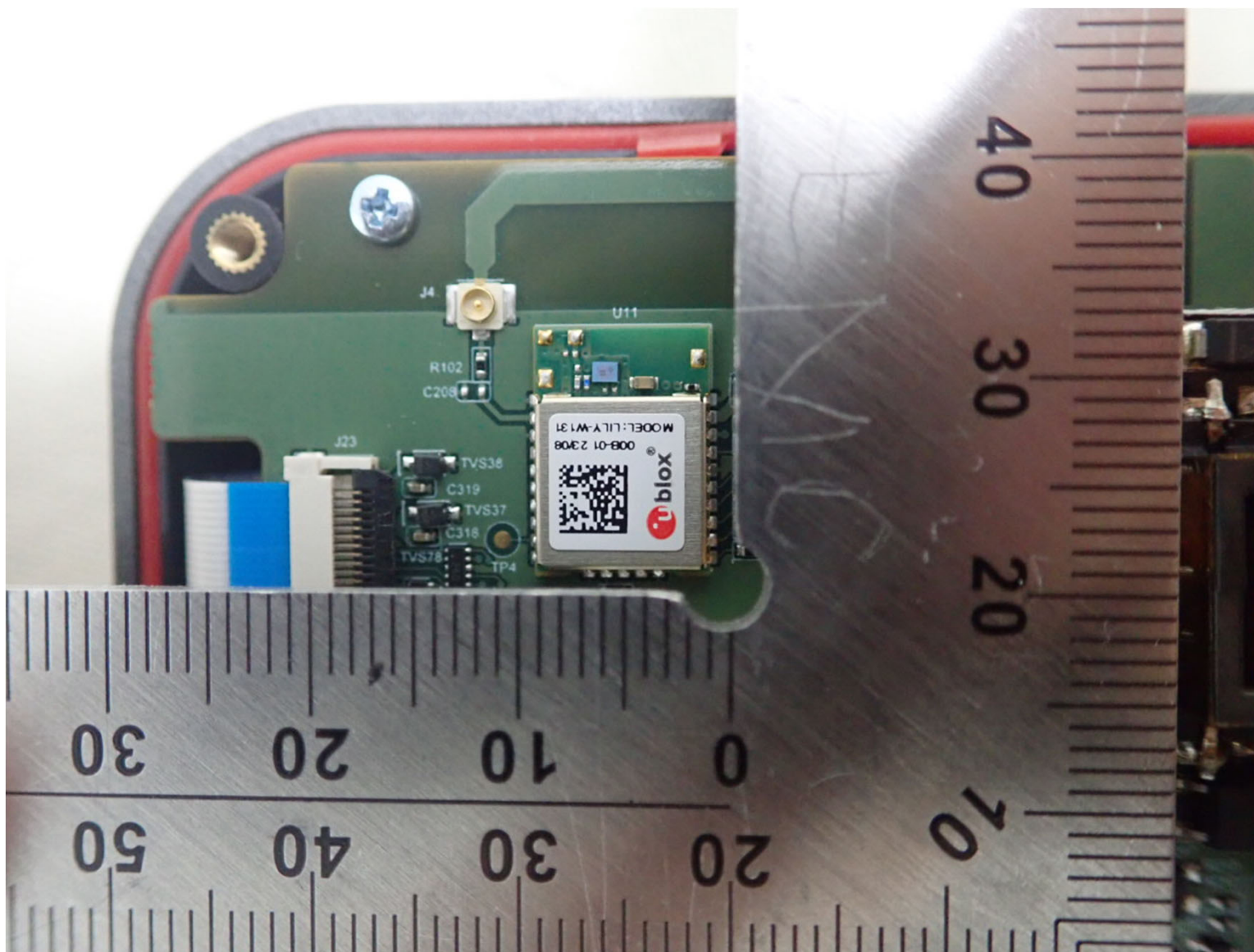
RF Module Front-1
