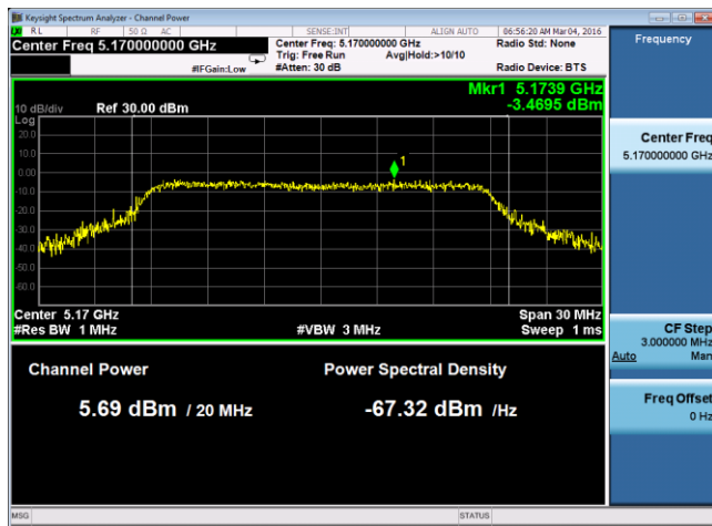
PSD - 20M 5170MHz Port A
