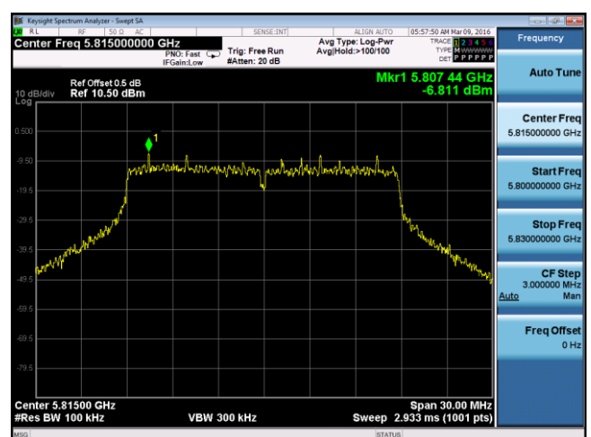
PSD - 20M 5815MHz Port B
