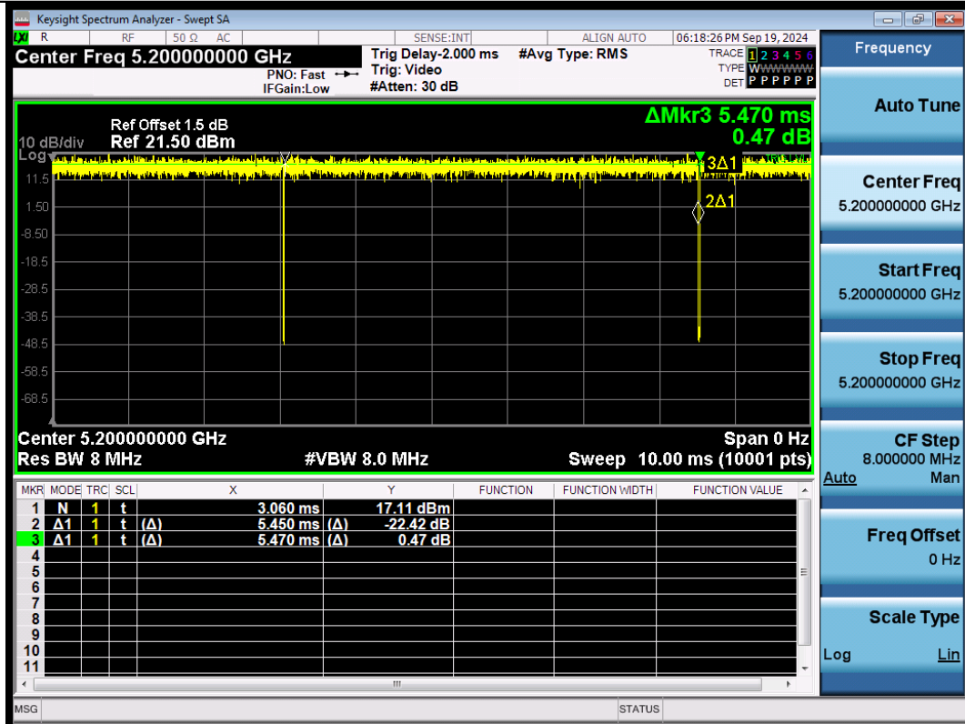
NTNV-11BE20SISO-Ant1-5200
