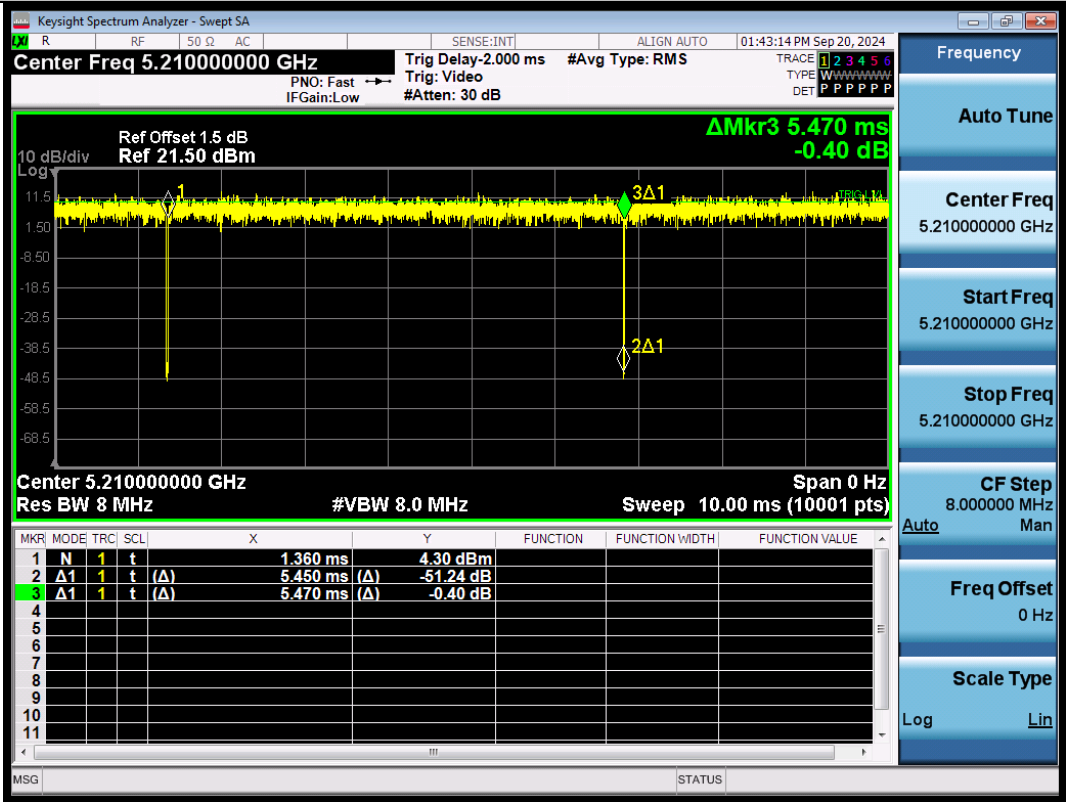
NTNV-11BE80SISO-Ant1-5210
