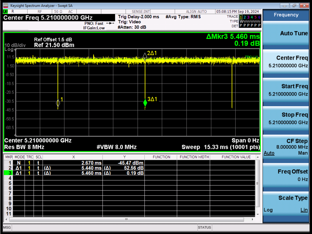
NTNV-11AX80SISO-Ant1-5210
