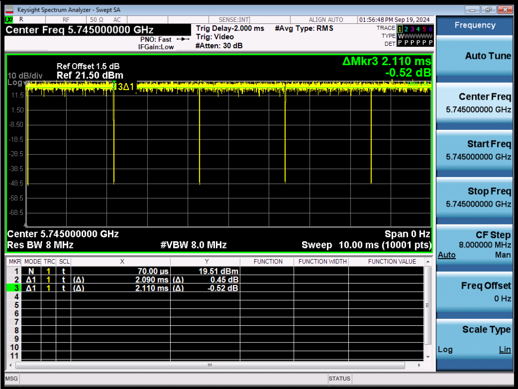
NTNV-11A-Ant1-5745
