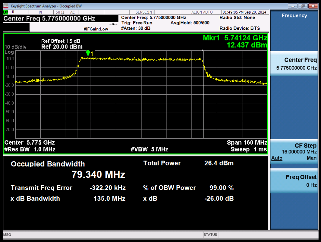
11BE80SISO-Ant1-5775
