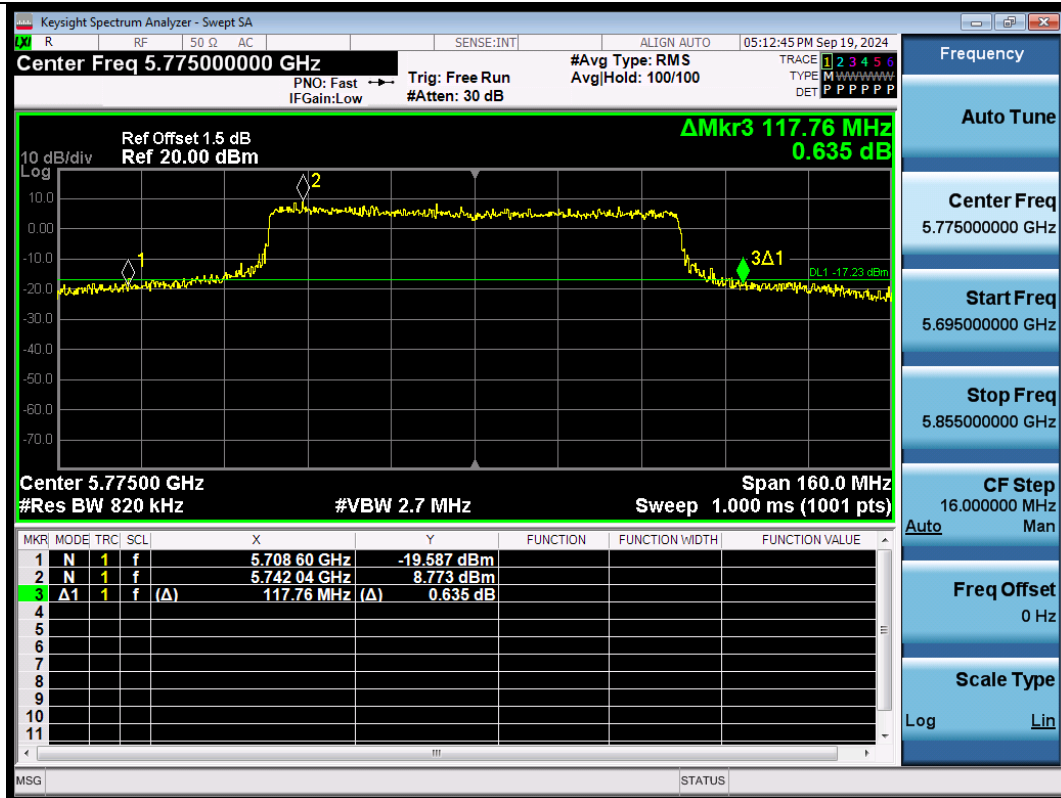
11AX80SISO-Ant1-5775
