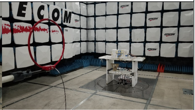
9kHz – 30MHz
