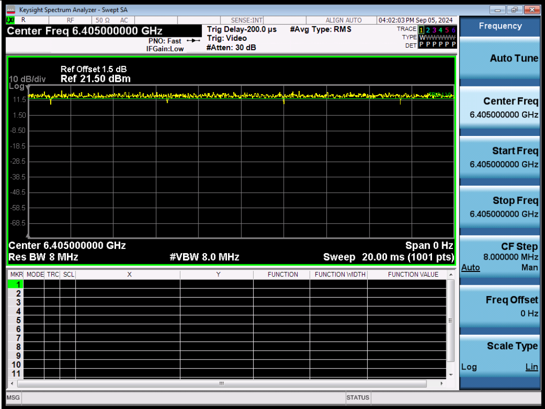
NTNV-11AX40SISO-Ant1-6405
