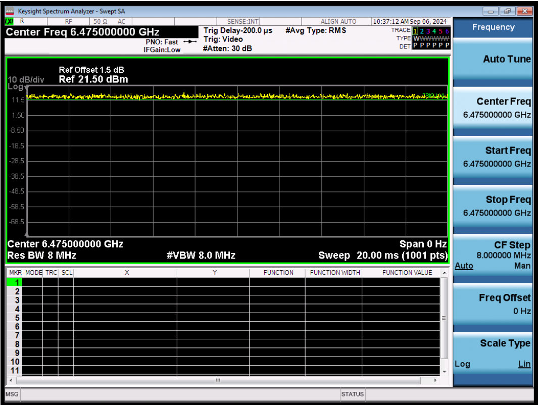
NTNV-11BE20SISO-Ant1-6475
