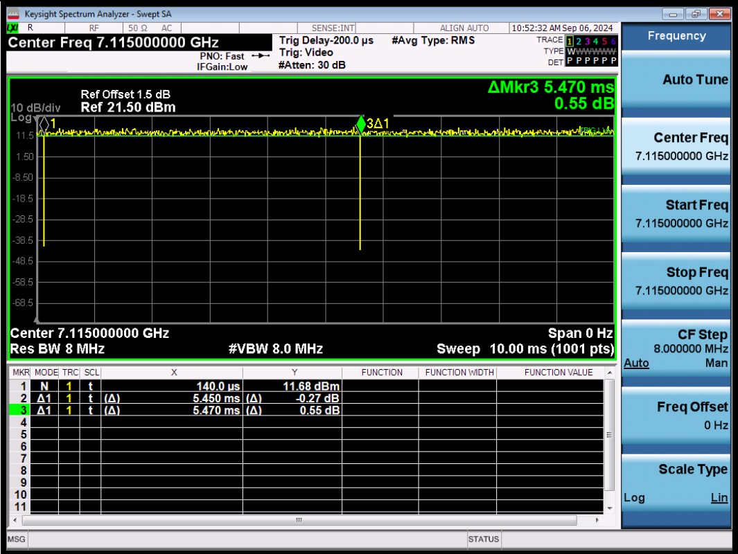
NTNV-11BE20SISO-Ant1-7115
