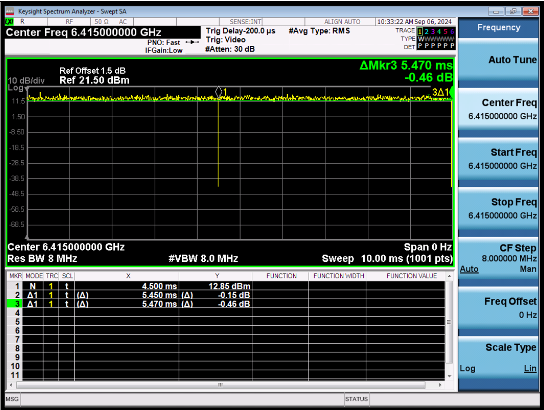
NTNV-11BE20SISO-Ant1-6415
