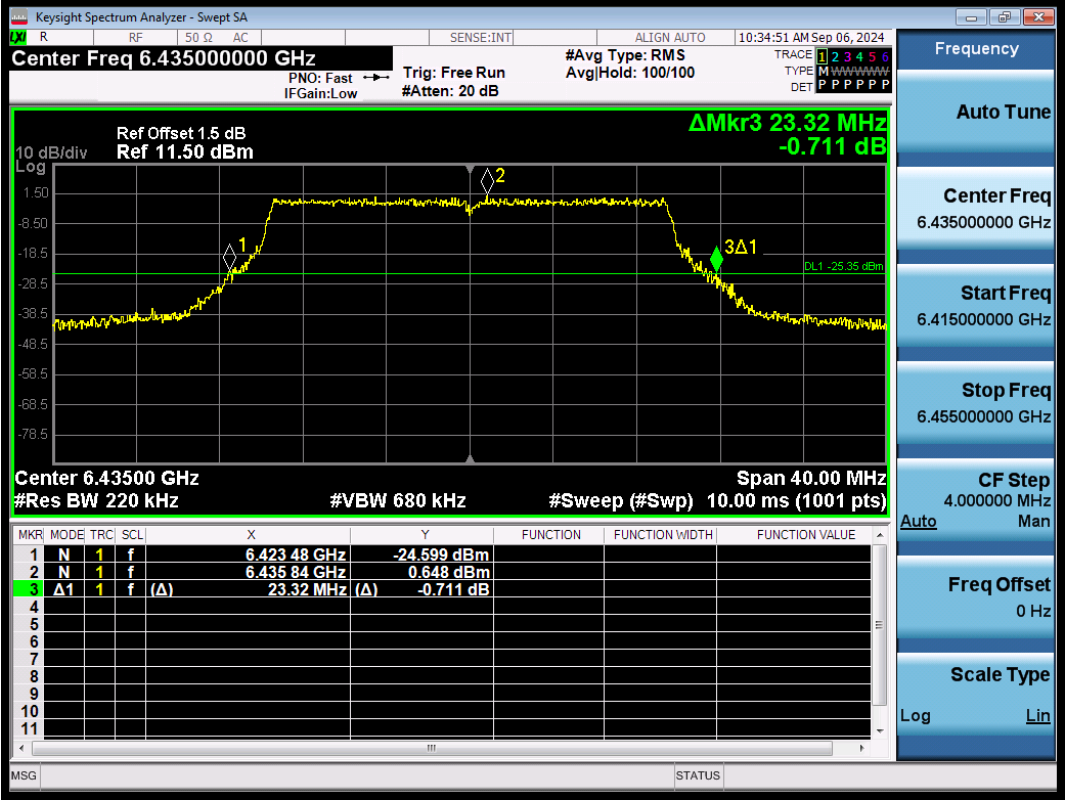
11BE20SISO-Ant1-6435
