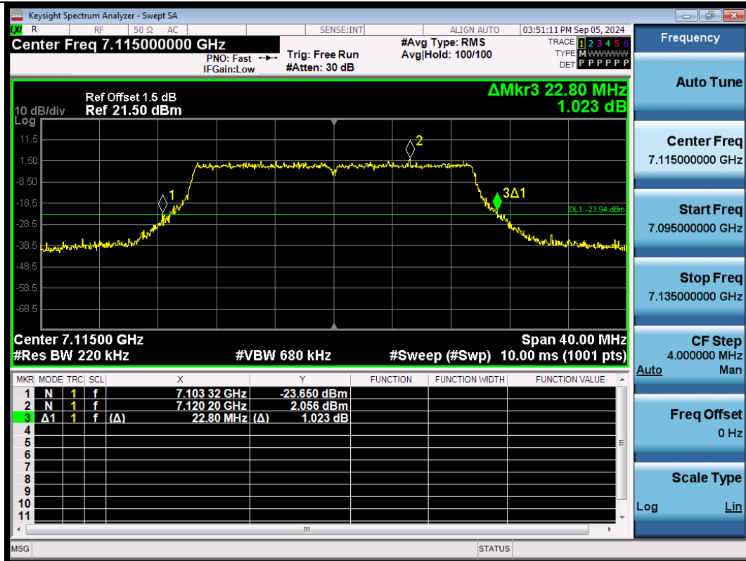
11AX20SISO-Ant1-7115
