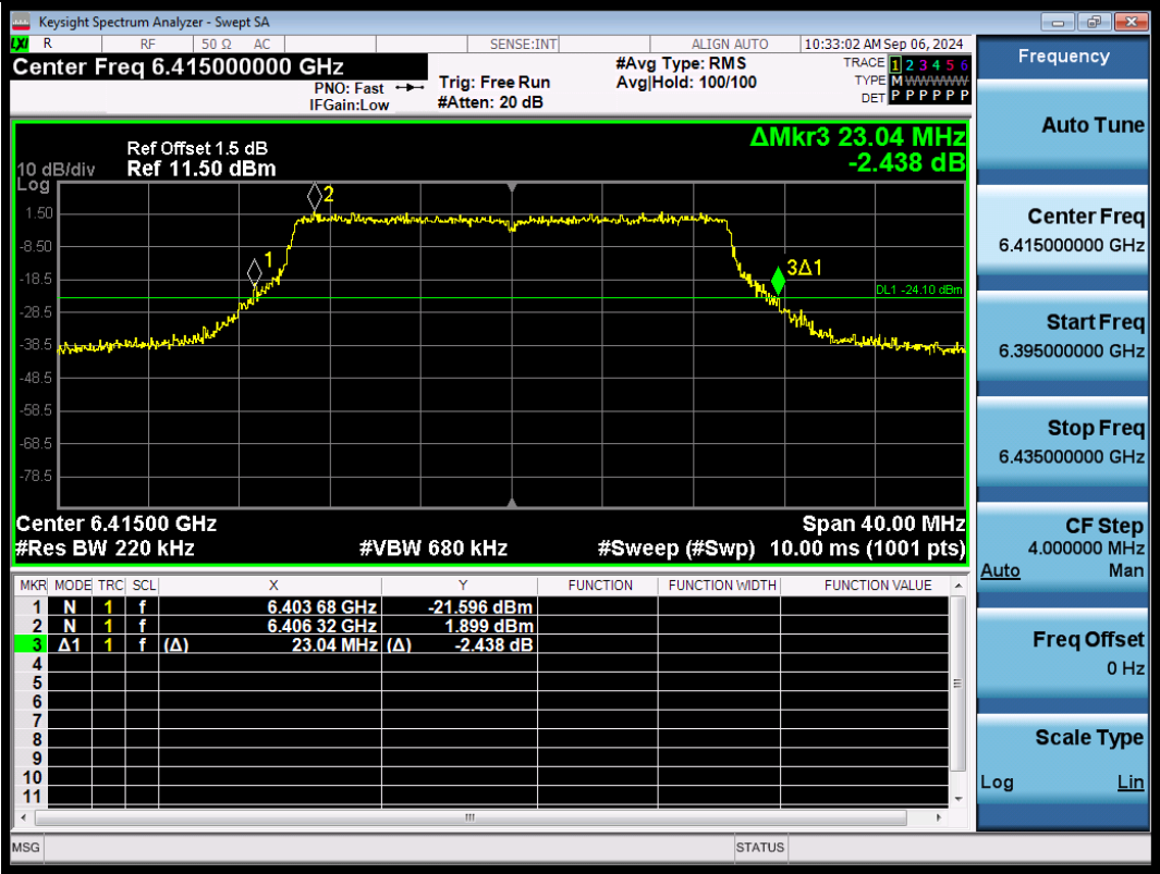
11BE20SISO-Ant1-6415
