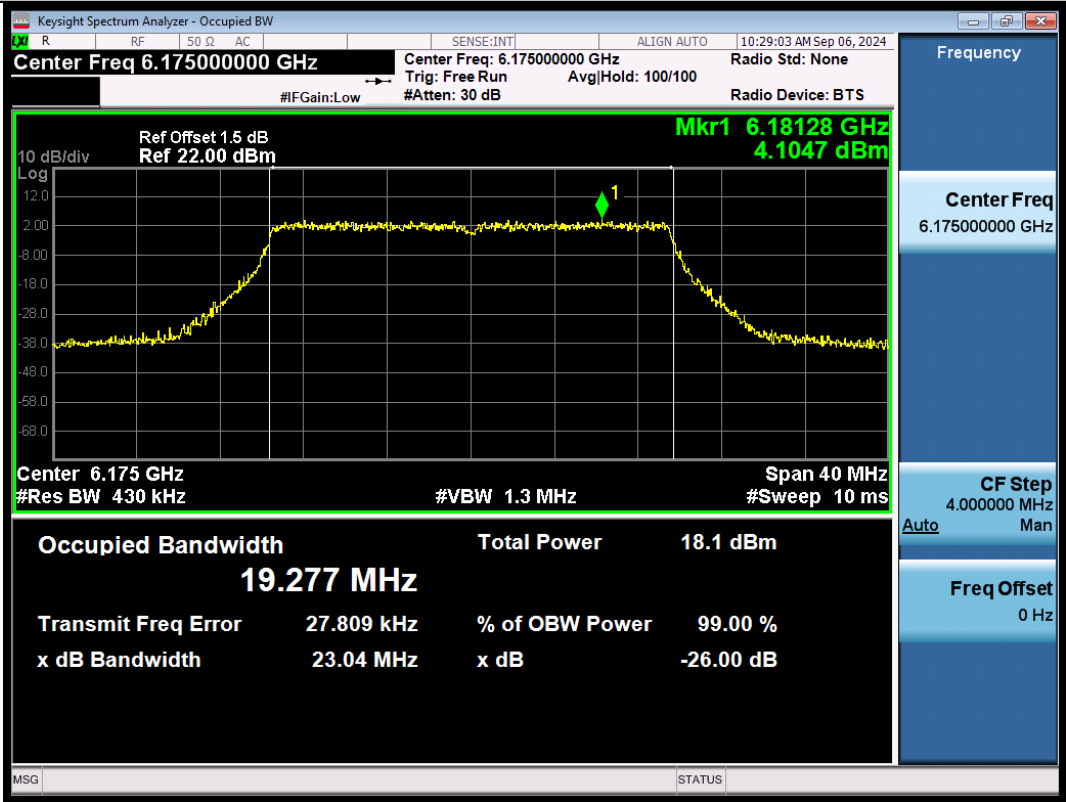
11BE20SISO-Ant1-6175-PASS
