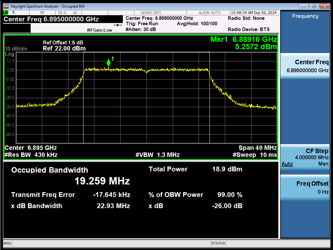
11BE20SISO-Ant1-6895-PASS
