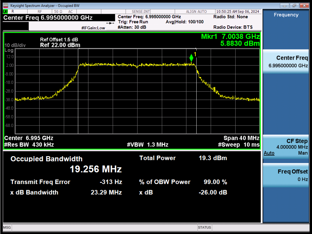
11BE20SISO-Ant1-6995-PASS
