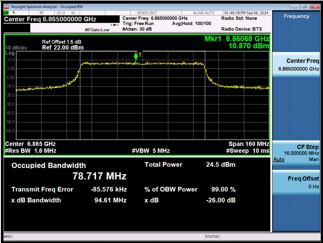
11BE80SISO-Ant1-6865-PASS
