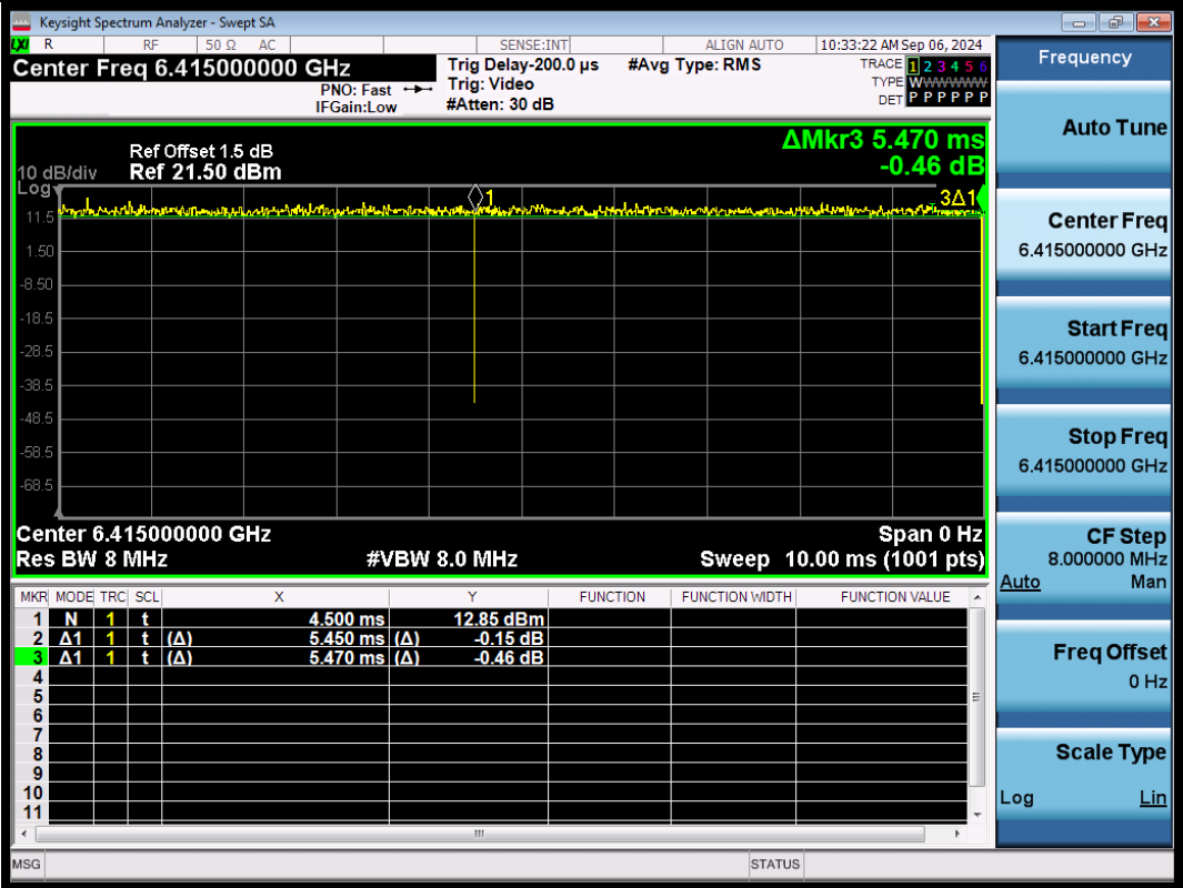
NTNV-11BE20SISO-Ant1-6415
