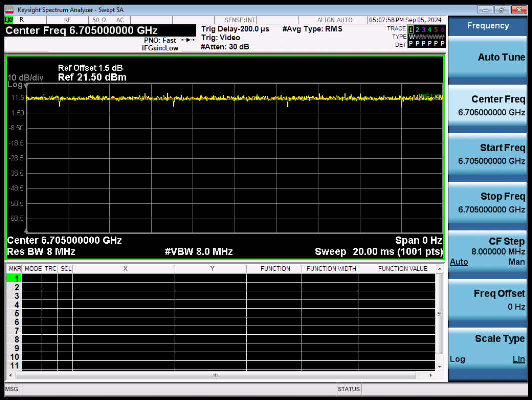
NTNV-11AX80SISO-Ant1-6705
