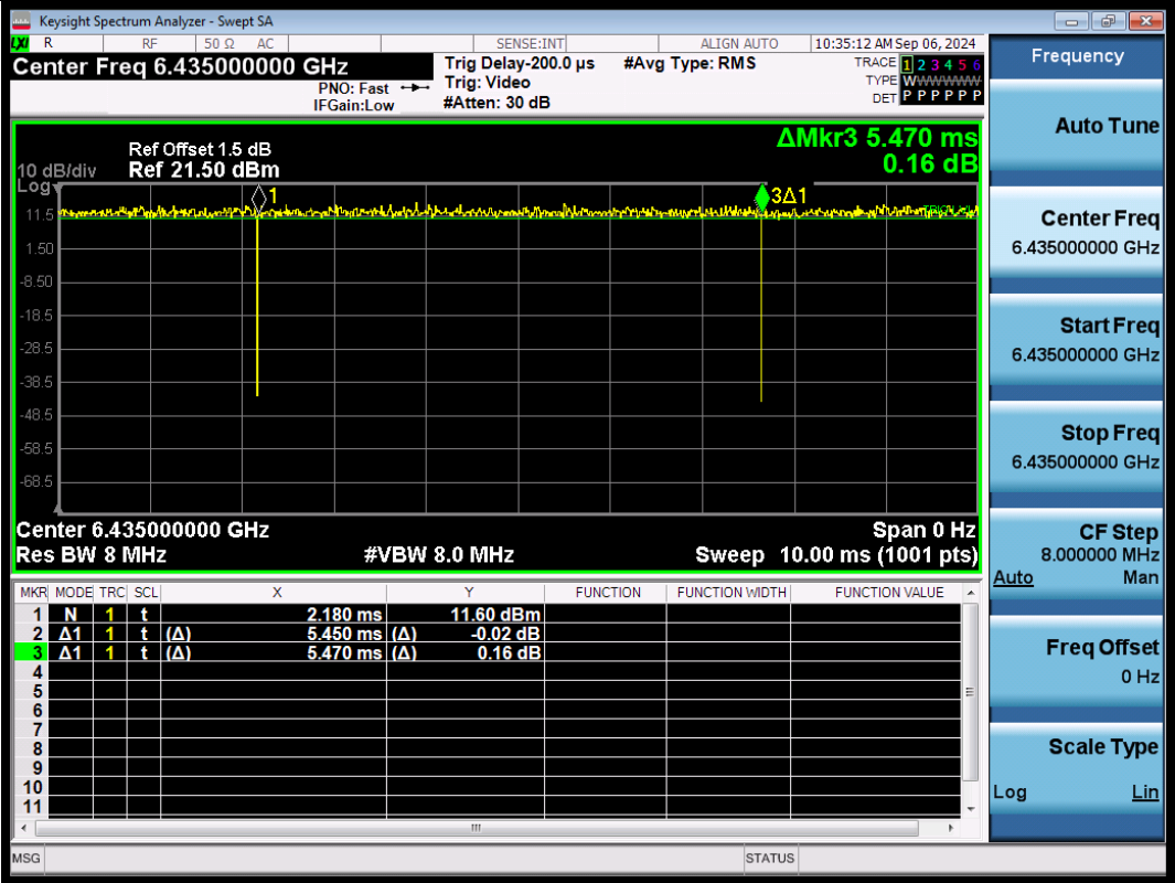
NTNV-11BE20SISO-Ant1-6435
