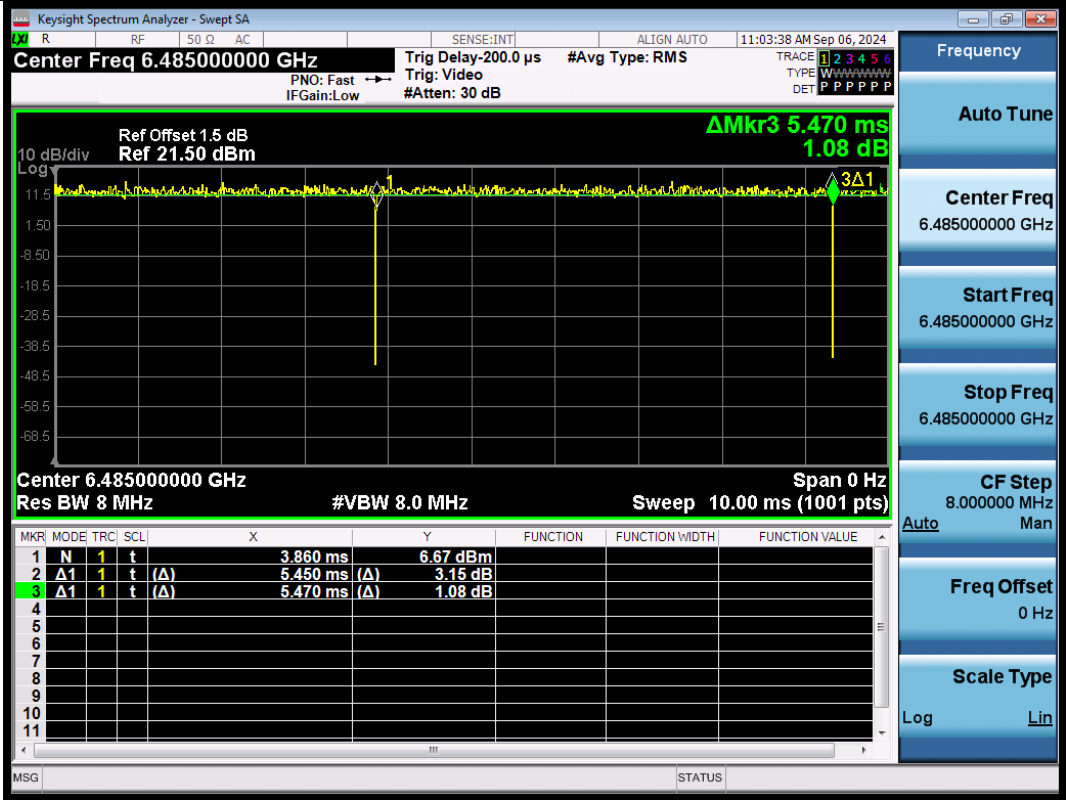
NTNV-11BE40SISO-Ant1-6485
