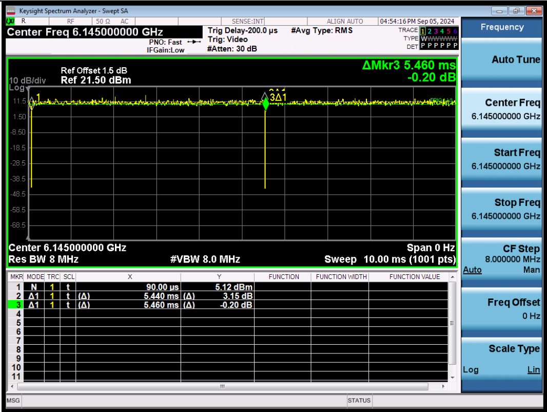
NTNV-11AX80SISO-Ant1-6145
