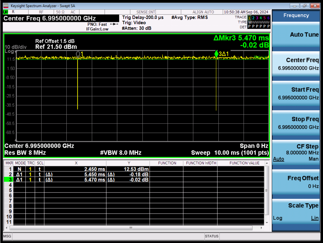
NTNV-11BE20SISO-Ant1-6995
