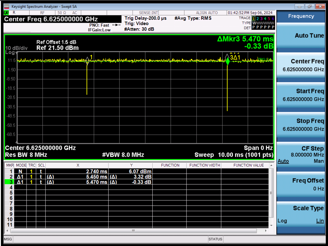
NTNV-11BE80SISO-Ant1-6625
