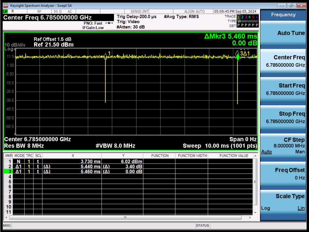
NTNV-11AX80SISO-Ant1-6785
