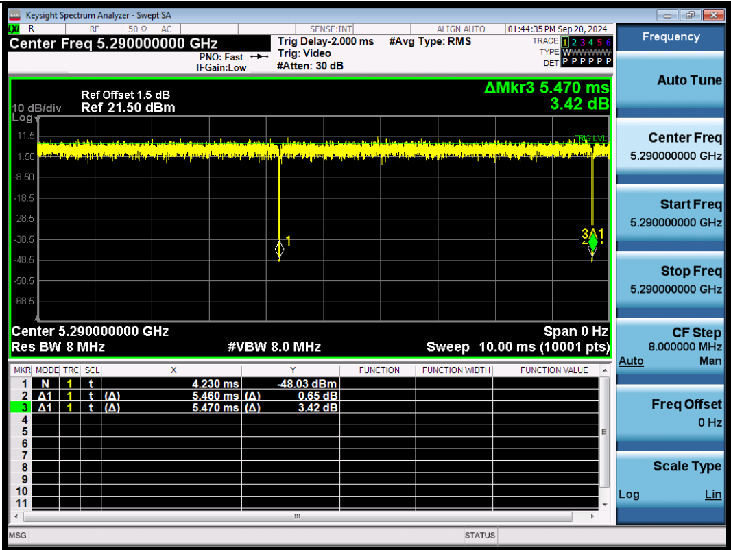
NTNV-11BE80SISO-Ant1-5290
