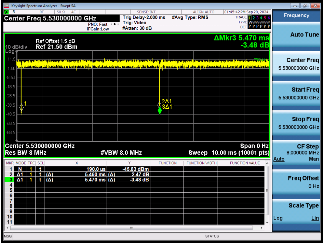
NTNV-11BE80SISO-Ant1-5530
