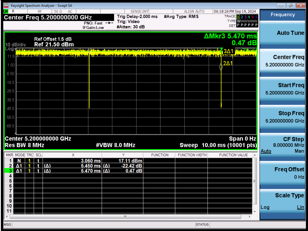
NTNV-11BE20SISO-Ant1-5200
