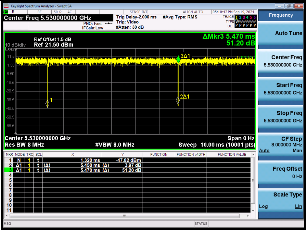
NTNV-11AX80SISO-Ant1-5530
