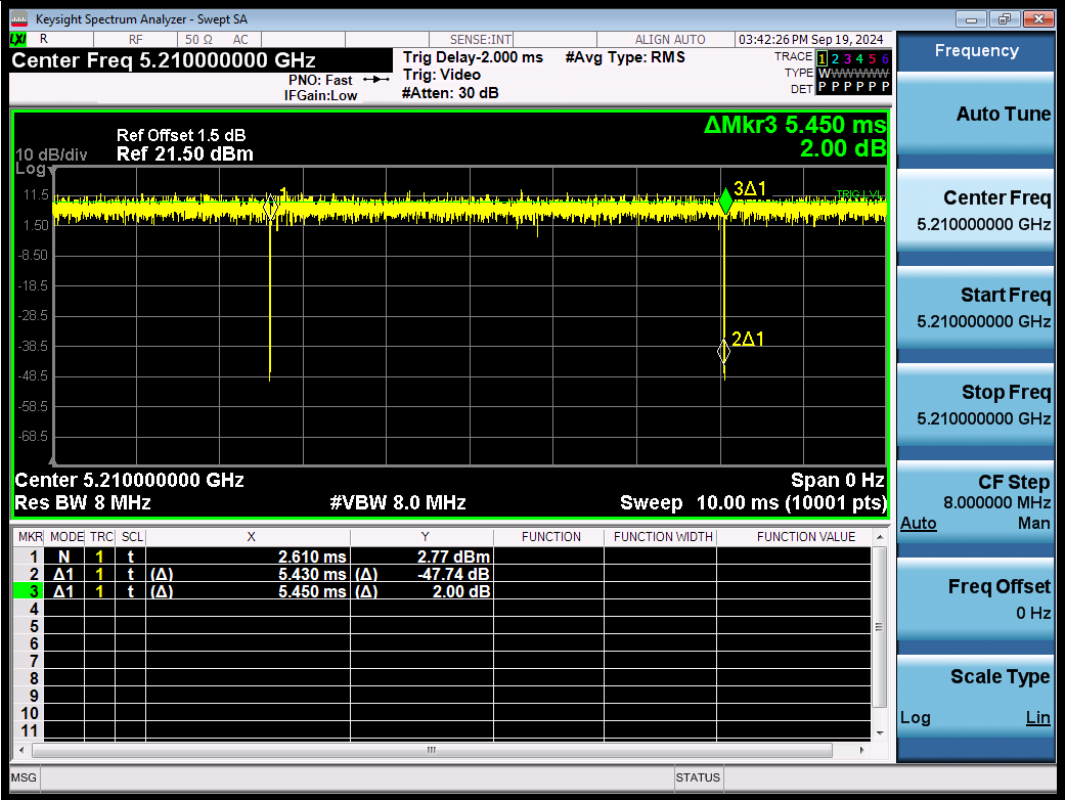
NTNV-11AC80SISO-Ant1-5210
