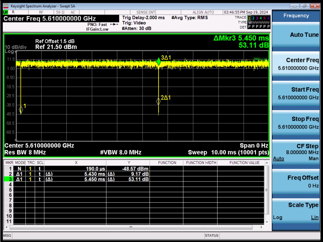
NTNV-11AC80SISO-Ant1-5610
