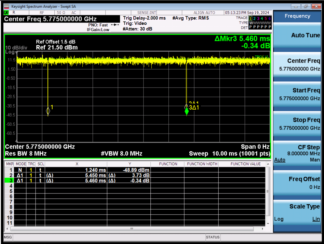
NTNV-11AX80SISO-Ant1-5775
