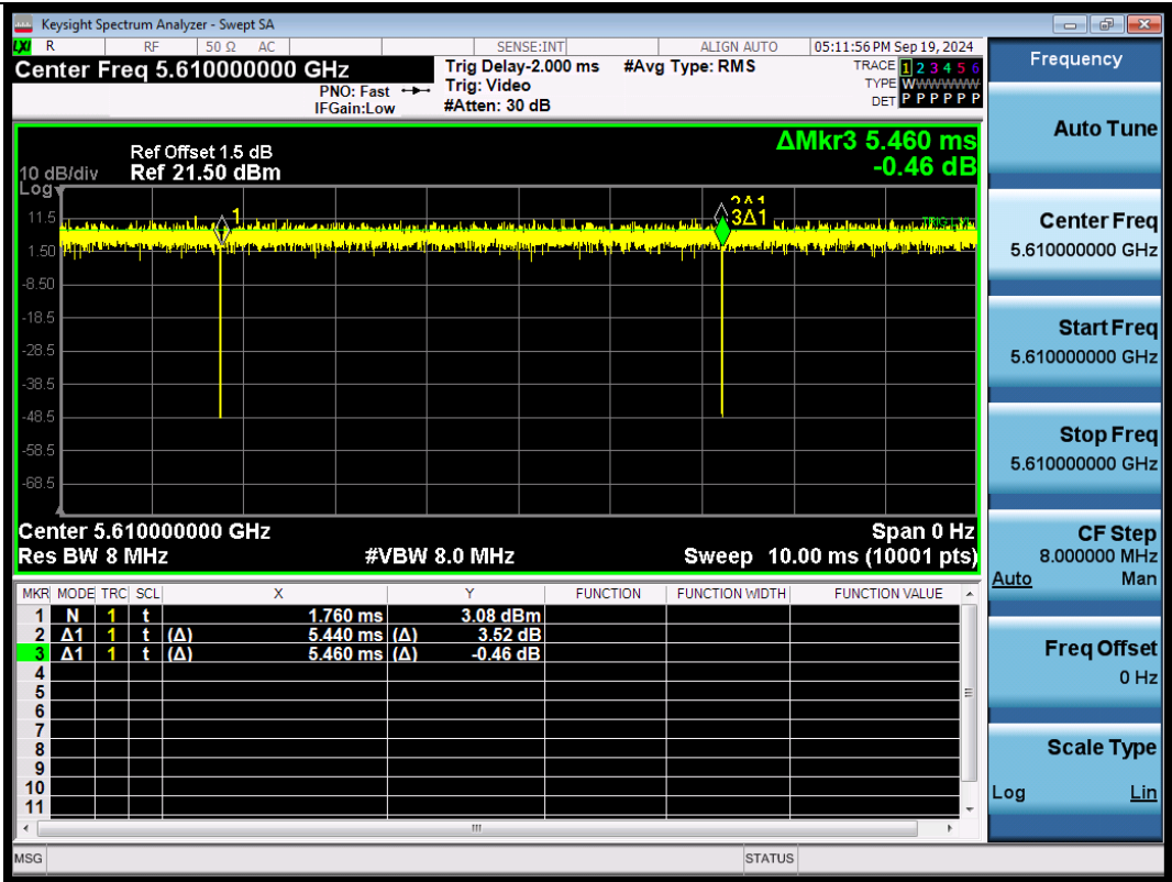
NTNV-11AX80SISO-Ant1-5610
