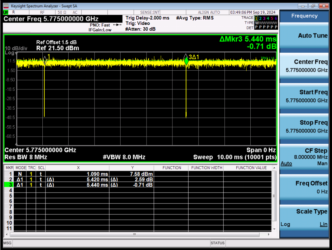
NTNV-11AC80SISO-Ant1-5775
