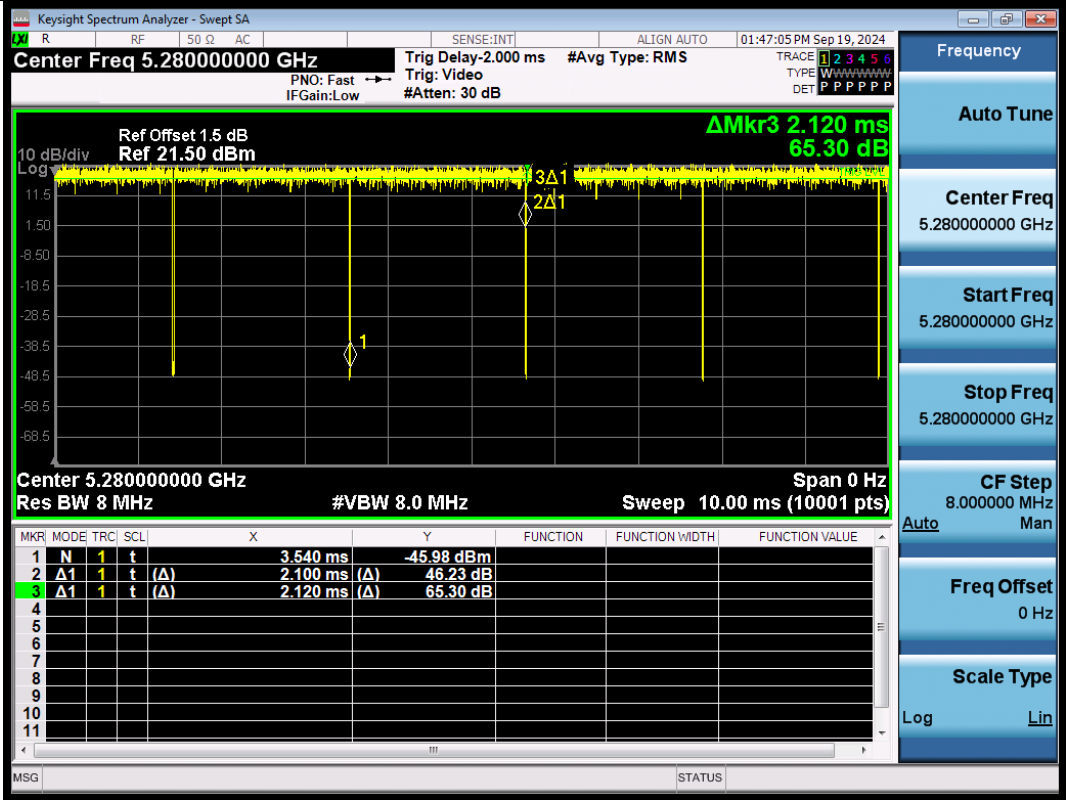
NTNV-11A-Ant1-5280
