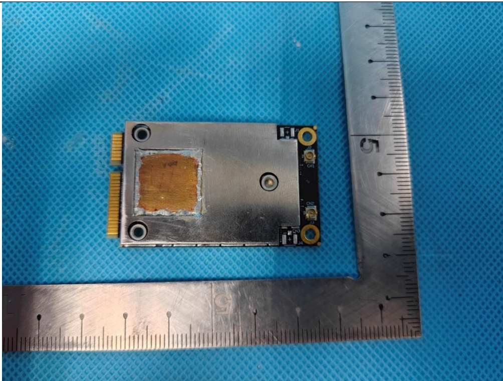
EUT Photo(6) - WLE7002E55
