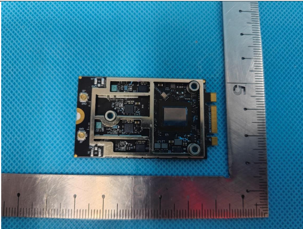
EUT Photo(4) - WLTB7002E55
