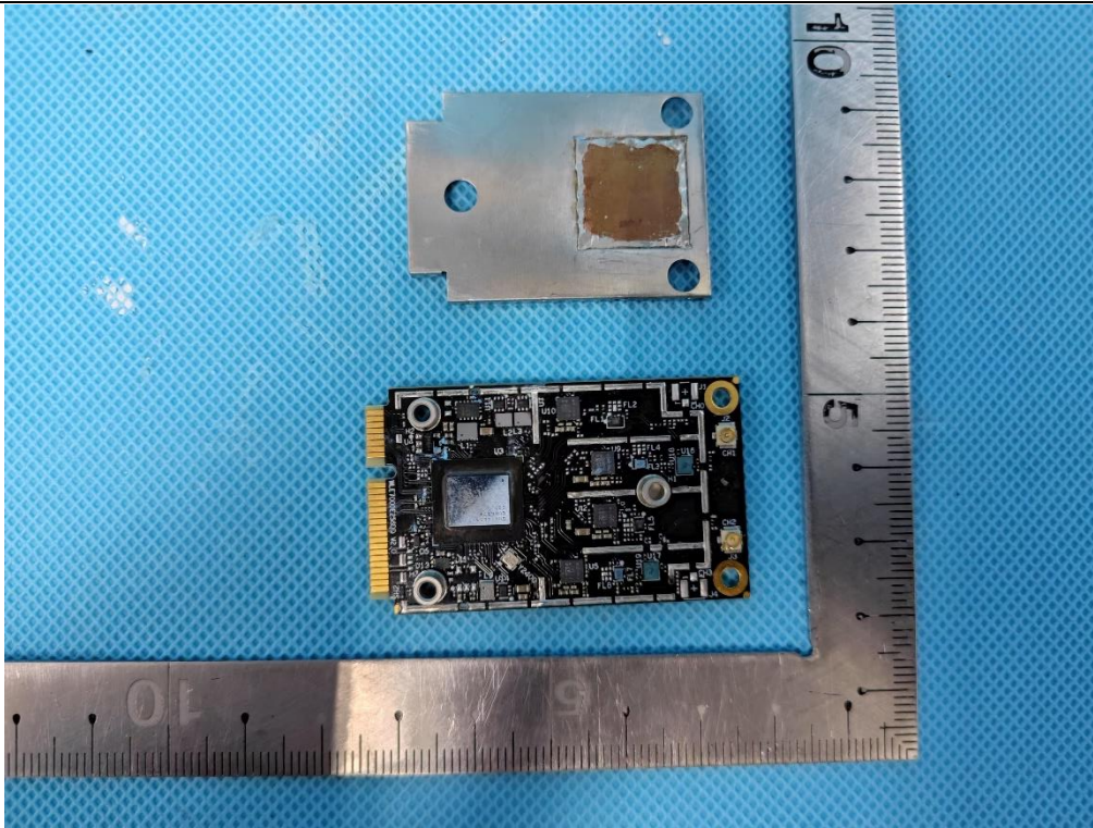
EUT Photo(8) - WLE7002E55
