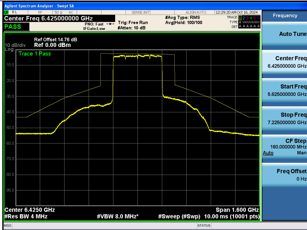
NTNV-11BE320SISO-Ant1-6425-PASS
