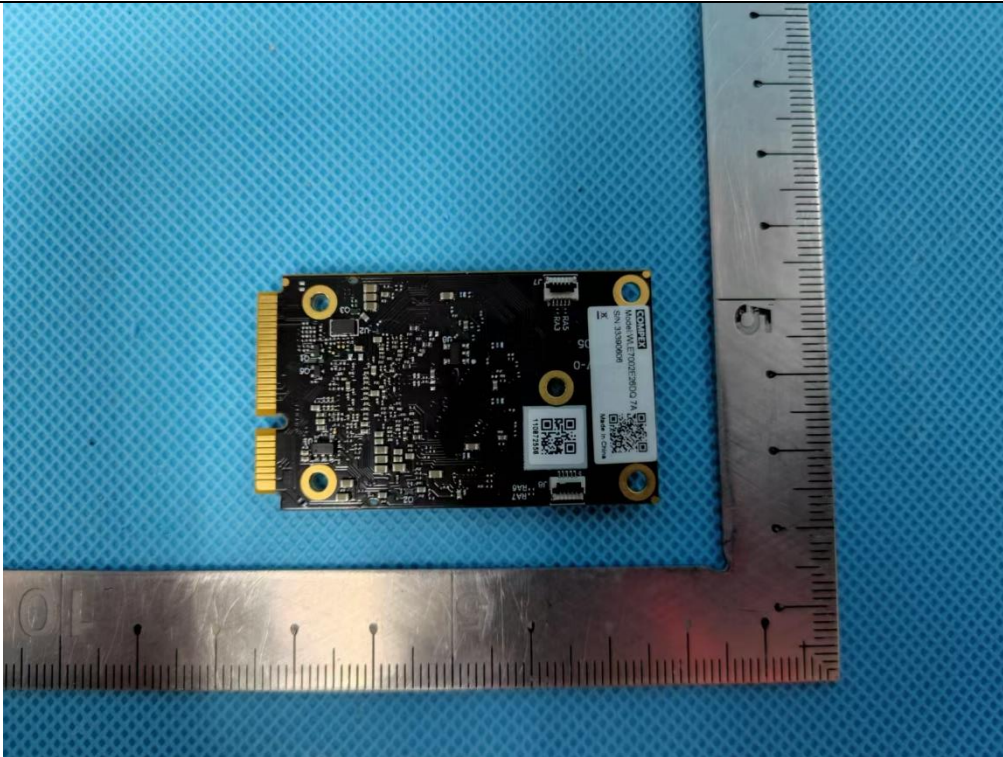
EUT Photo(8) - WLE7002E26
