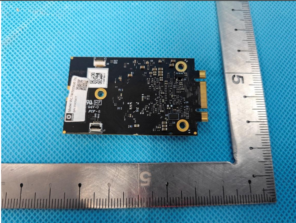
EUT Photo(4) - WLTB7002E26
