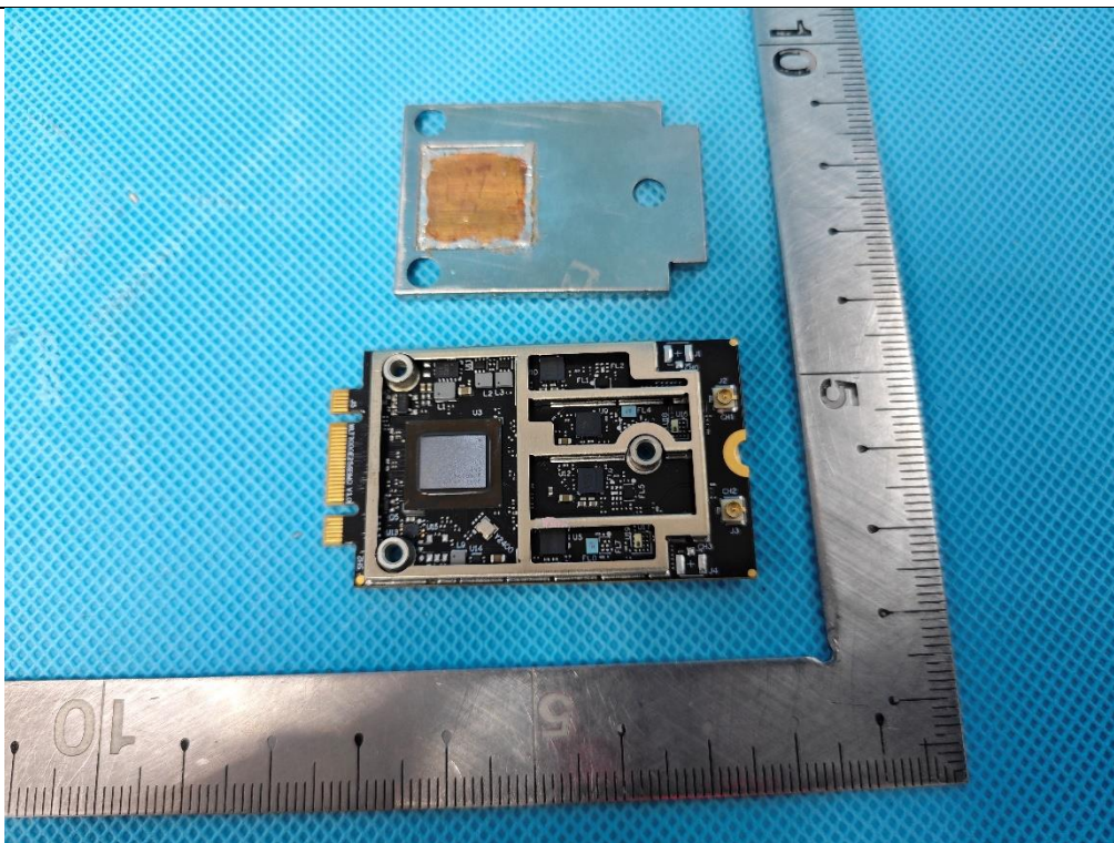
EUT Photo(2) - WLTB7002E26
