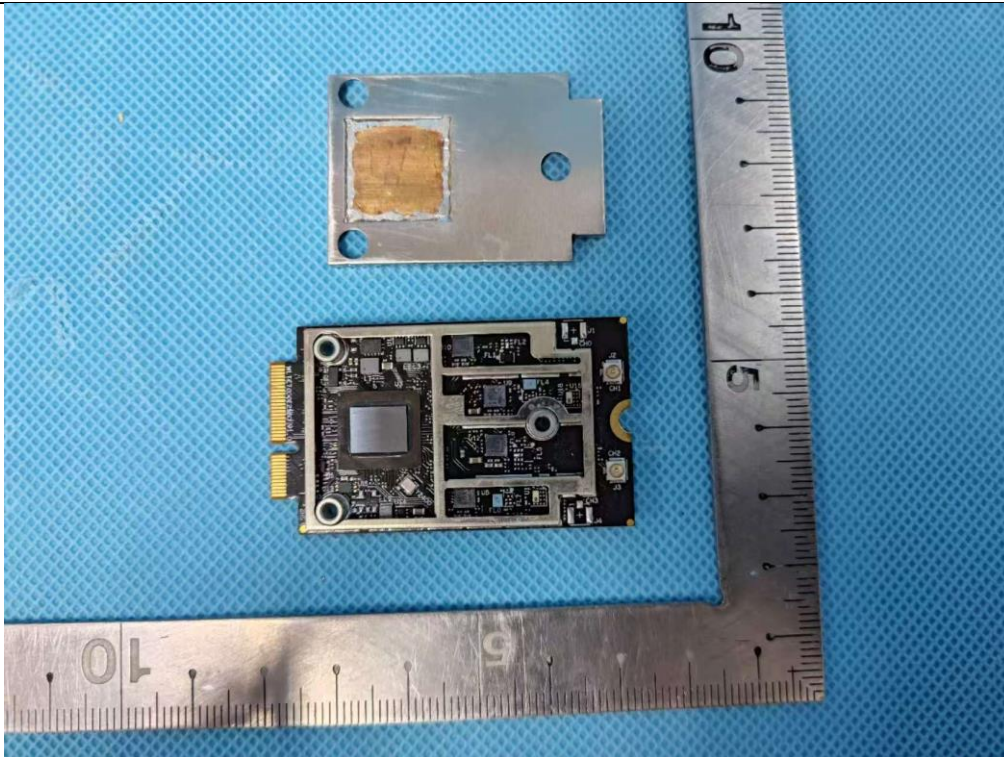
EUT Photo(10) - WLTE7002E26
