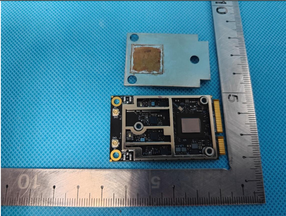
EUT Photo(6) - WLE7002E26
