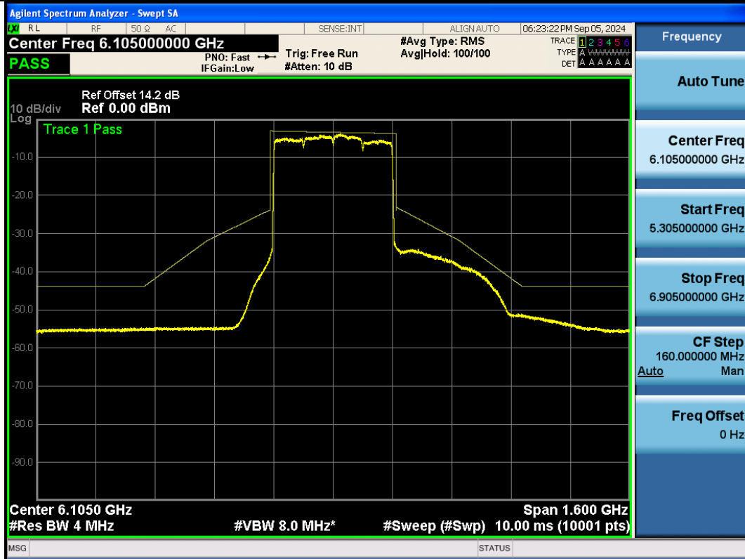
NTNV-11BE320SISO-Ant1-6105-PASS
