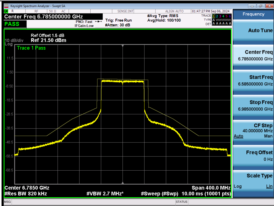
NTNV-11BE80SISO-Ant1-6785-PASS
