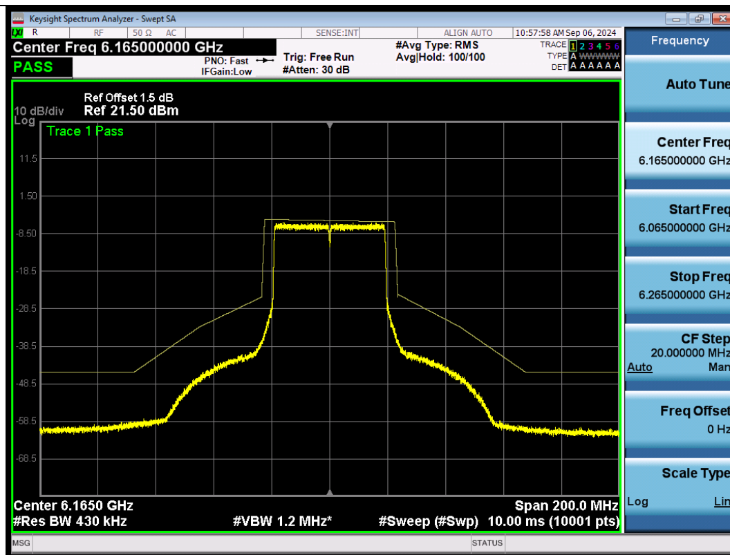
NTNV-11BE40SISO-Ant1-6165-PASS
