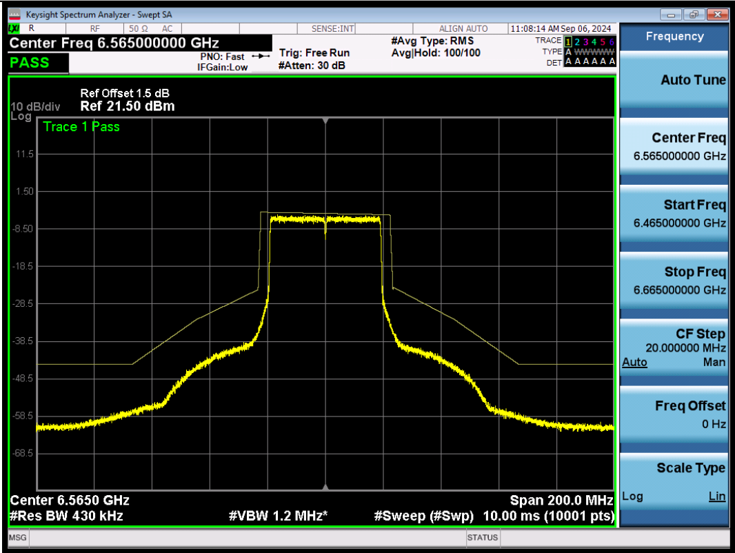
NTNV-11BE40SISO-Ant1-6565-PASS
