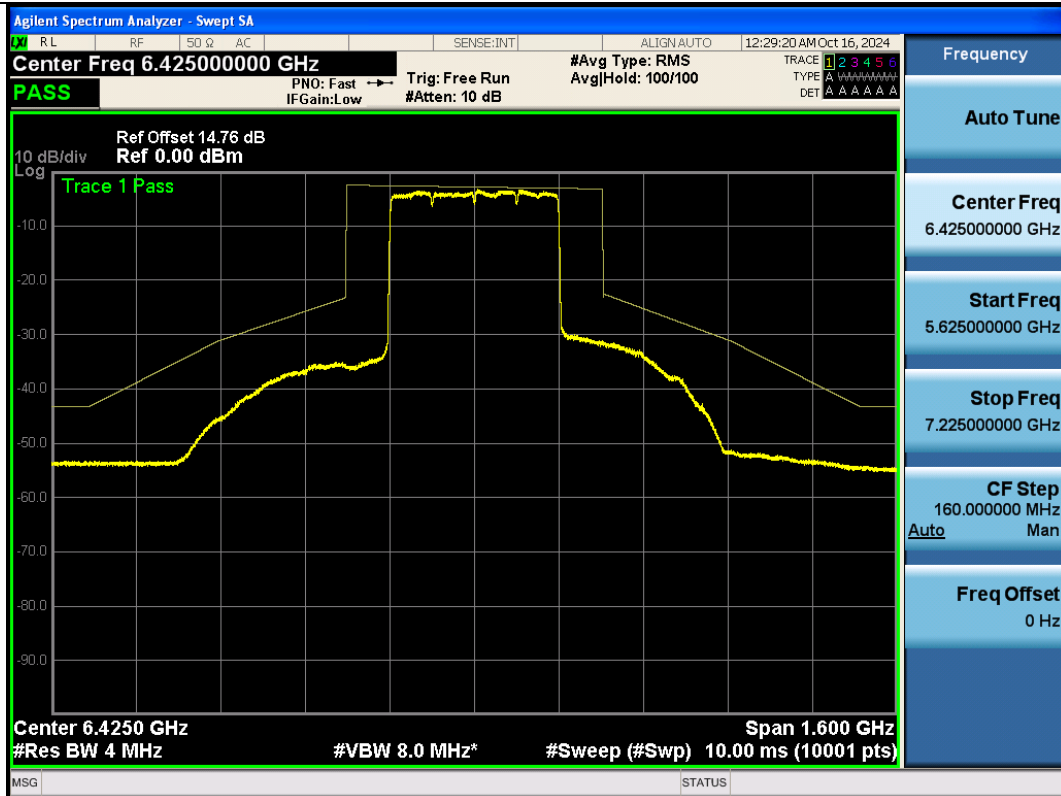
NTNV-11BE320SISO-Ant1-6425-PASS
