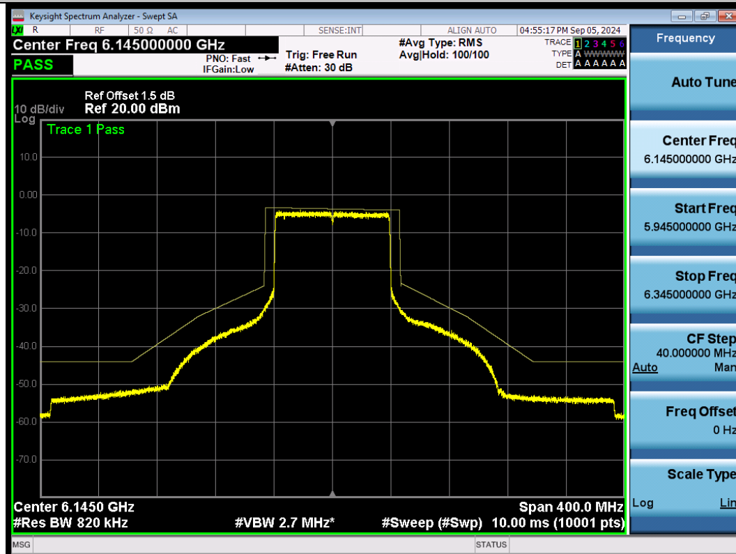
NTNV-11AX80SISO-Ant1-6145-PASS
