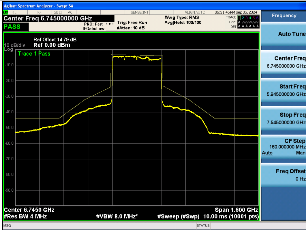
NTNV-11BE320SISO-Ant1-6745-PASS
