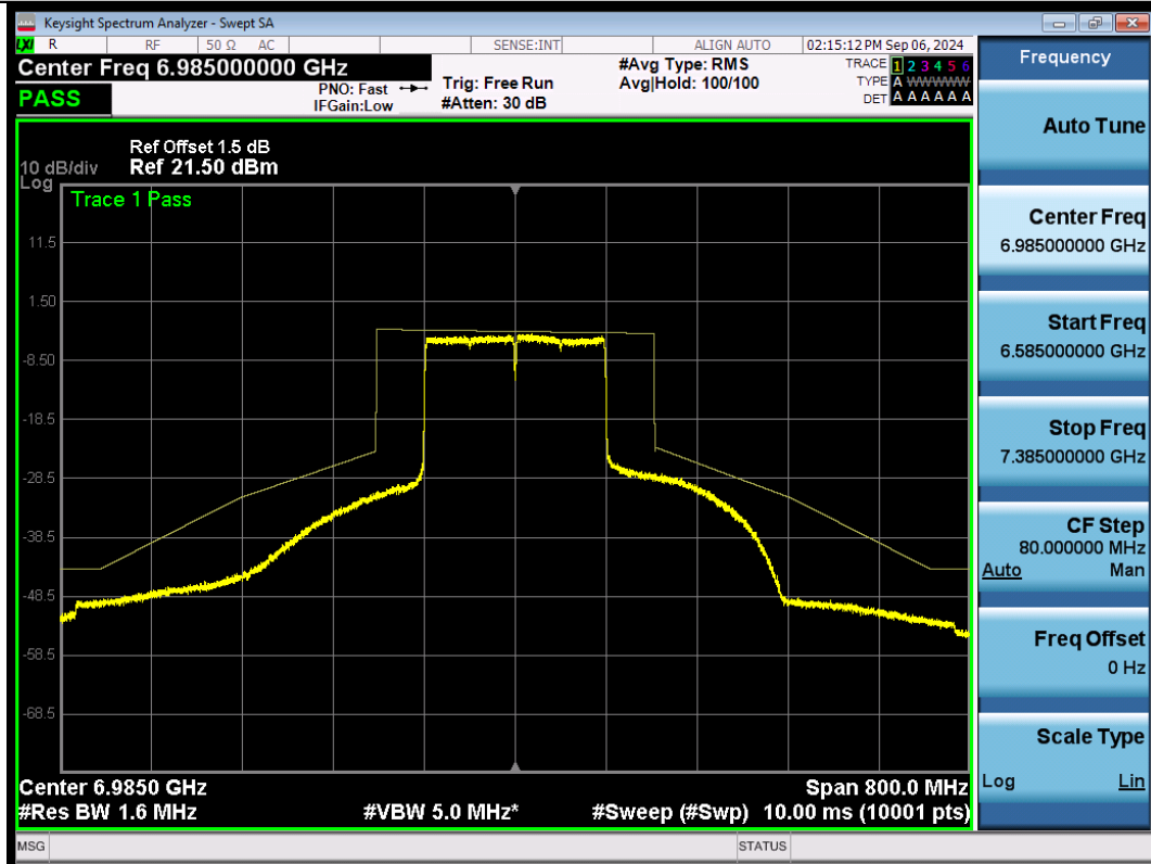
NTNV-11BE160SISO-Ant1-6985-PASS
