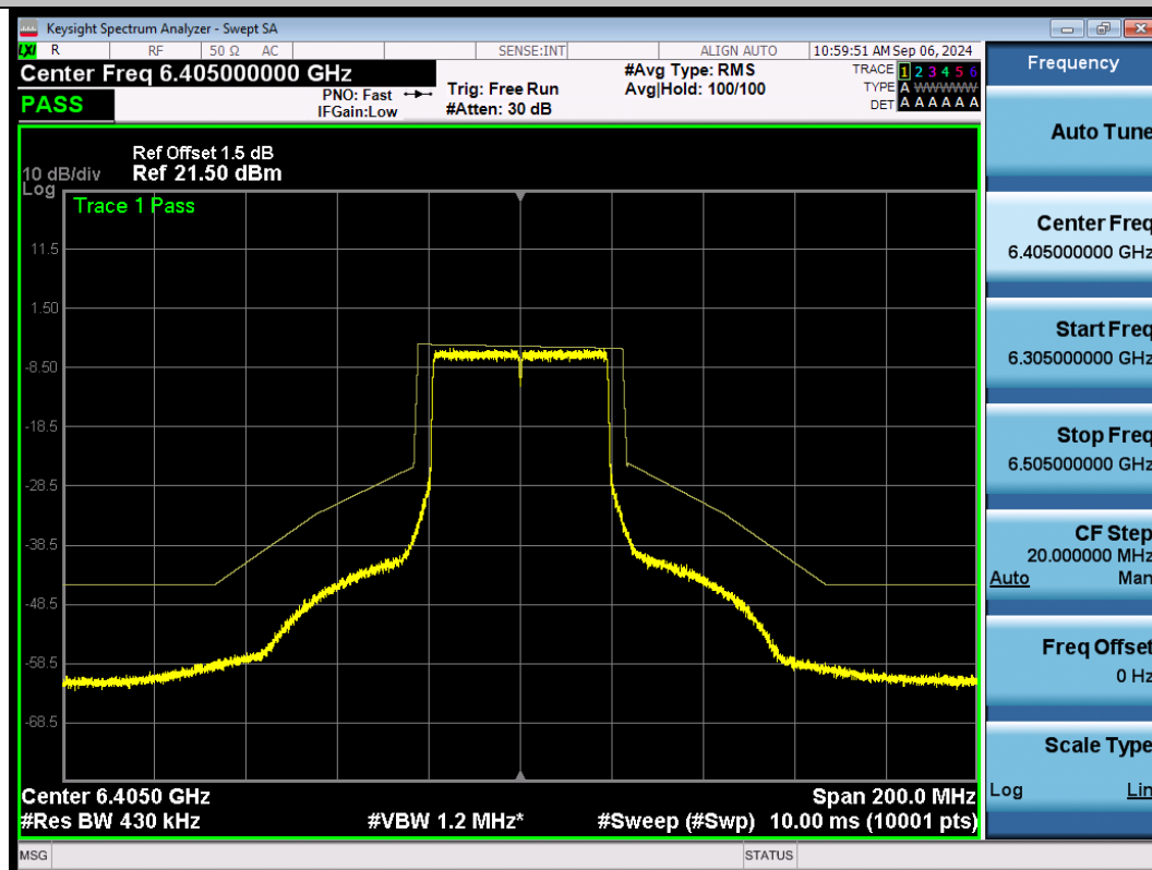
NTNV-11BE40SISO-Ant1-6405-PASS
