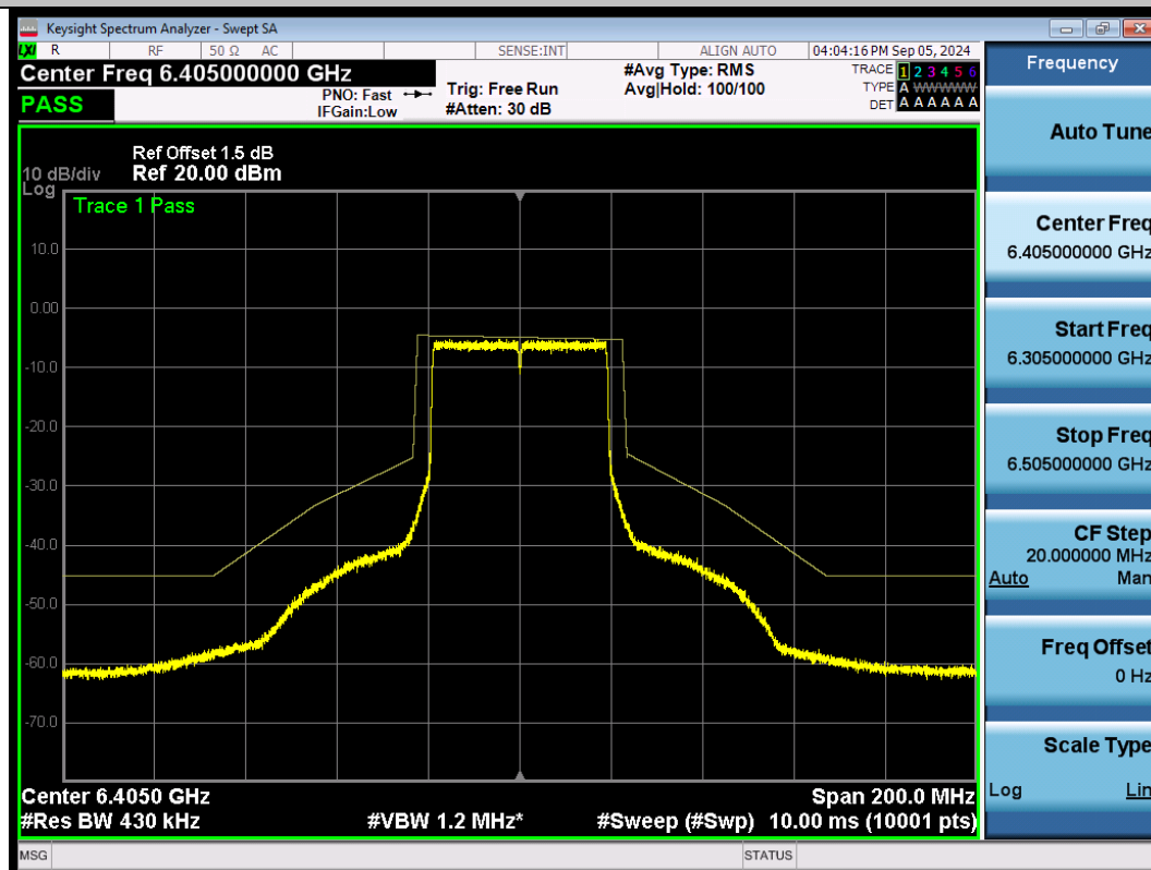
NTNV-11AX40SISO-Ant1-6405-PASS
