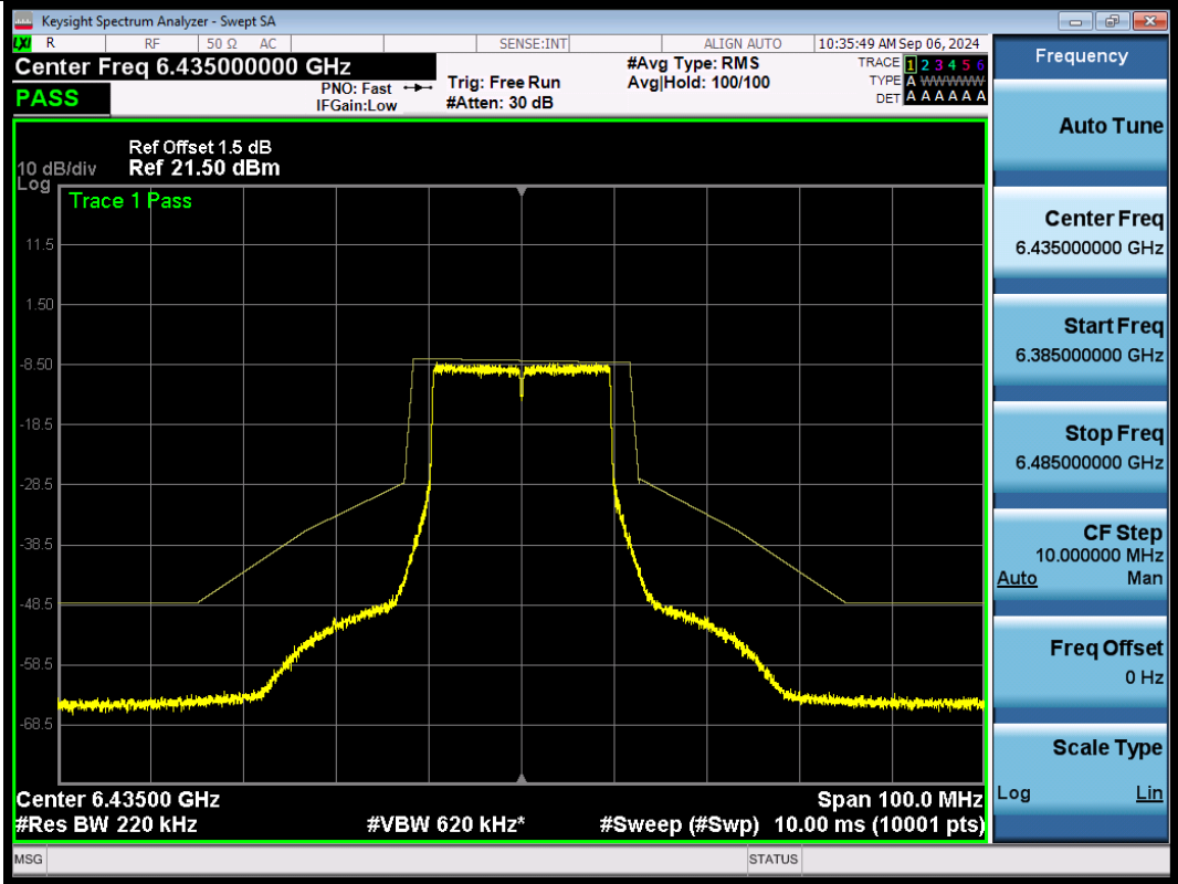
NTNV-11BE20SISO-Ant1-6435-PASS
