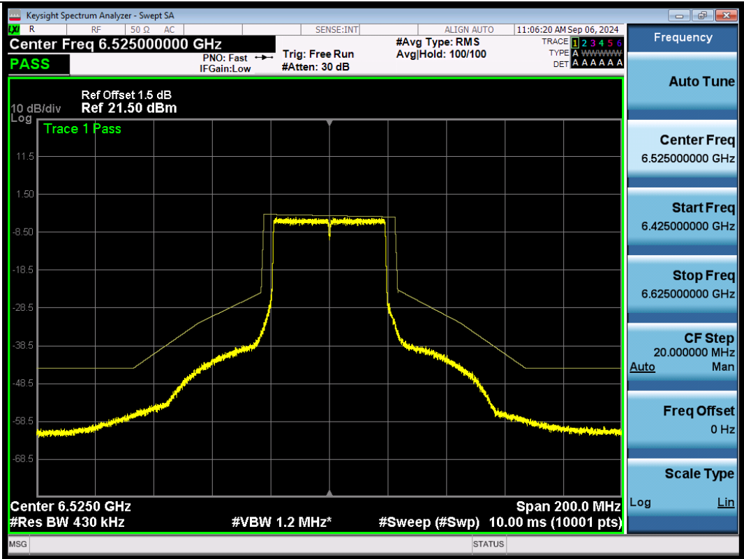
NTNV-11BE40SISO-Ant1-6525-PASS
