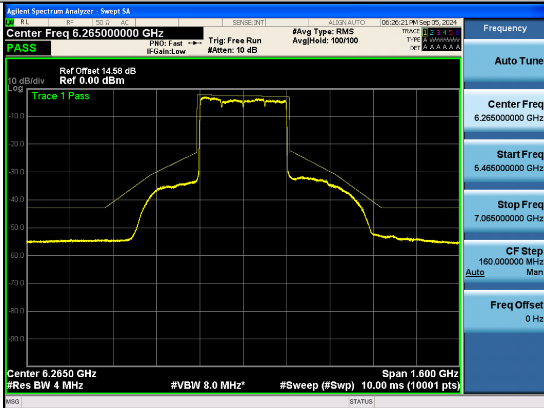
NTNV-11BE320SISO-Ant1-6265-PASS
