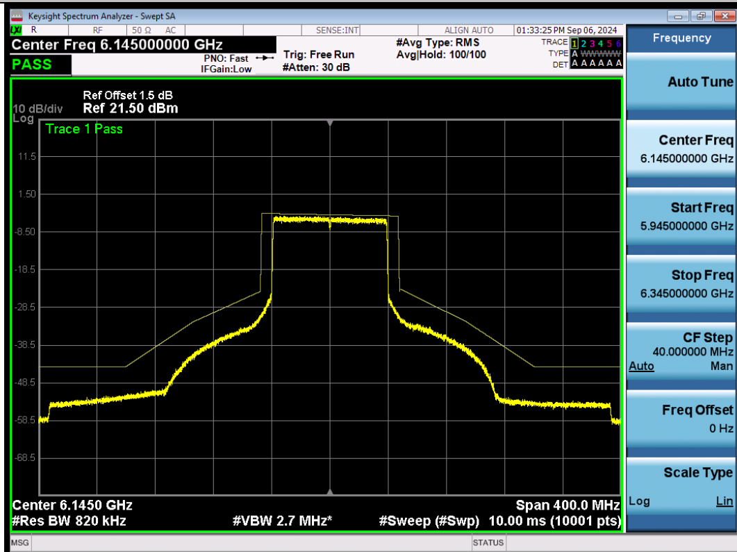
NTNV-11BE80SISO-Ant1-6145-PASS
